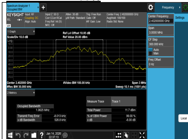
IC OBW_BLE 1M LowCH00-2402MHz
