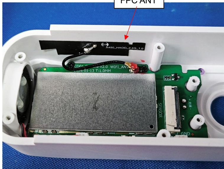
FPC ANT
