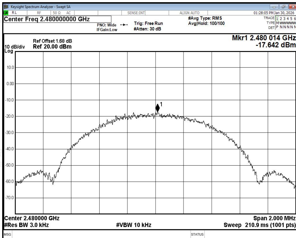
PSD NVNT BLE 1M 2480MHz Ant1
