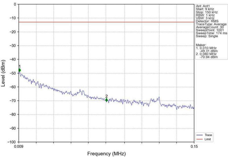
Band4 1.4MHz 16QAM LCH 1710.7MHz RB 1 0 NTV
