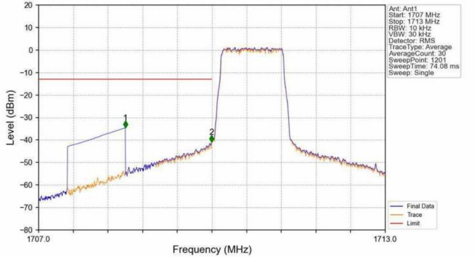
Band4 1.4MHz 16QAM LCH 1710.7MHz RB 6 0 NTV
