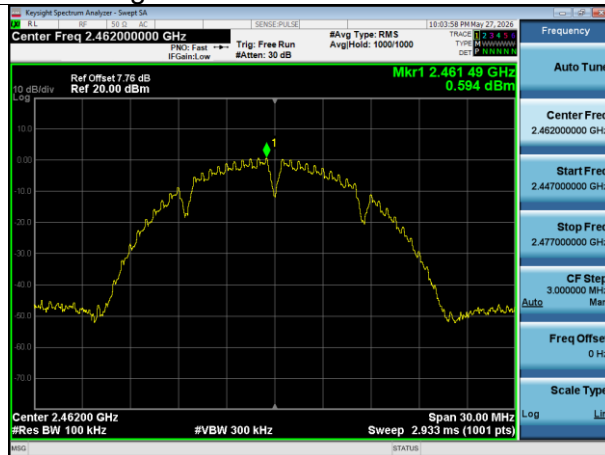
Band Edge NVNT b 2462MHz Ant1 Ref
