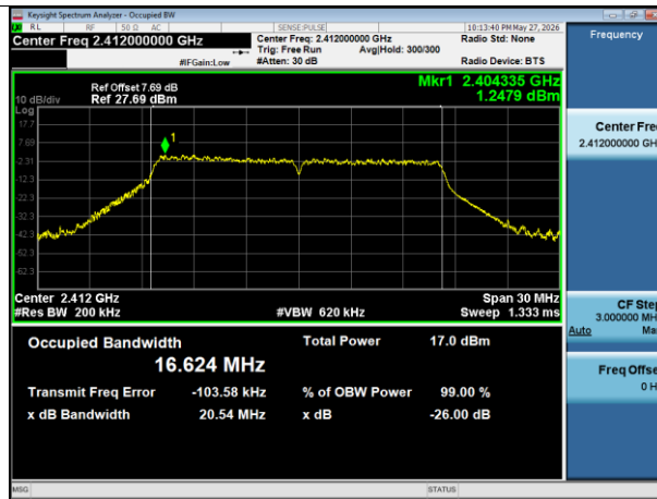
OBW NVNT g 2412MHz Ant1
