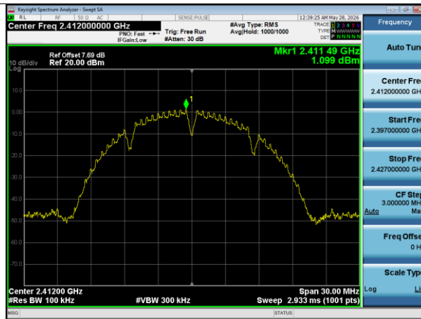
Band Edge NVNT b 2412MHz Ant1 Ref
