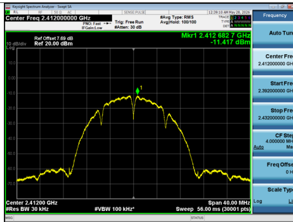
PSD NVNT b 2412MHz Ant1
