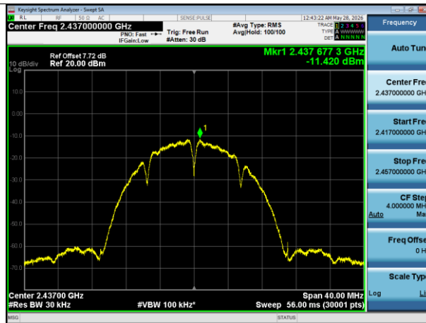
PSD NVNT b 2437MHz Ant1
