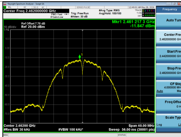
PSD NVNT b 2462MHz Ant1
