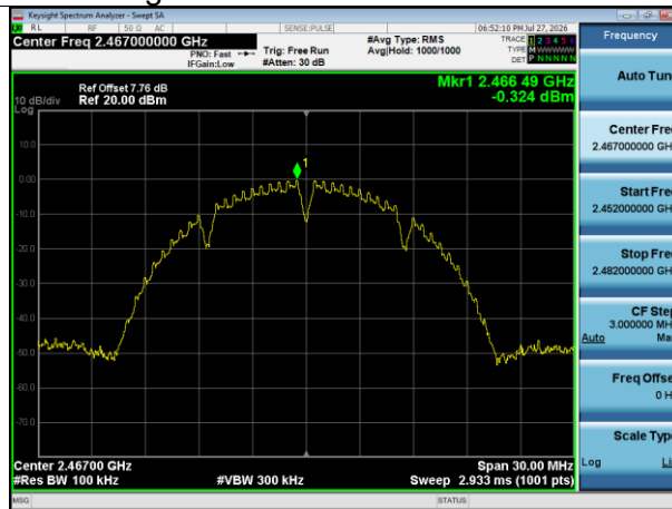
Band Edge NVNT b 2467MHz Ant1 Ref
