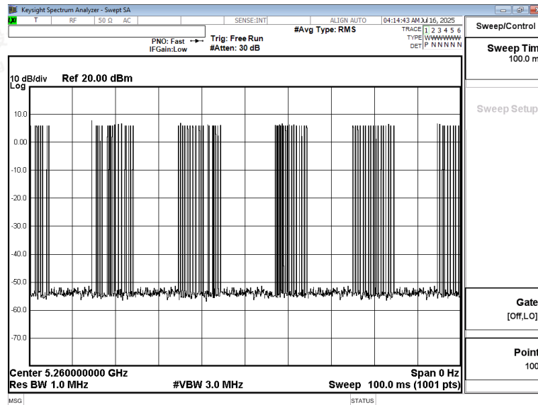
IEEE 802.11n HT20
