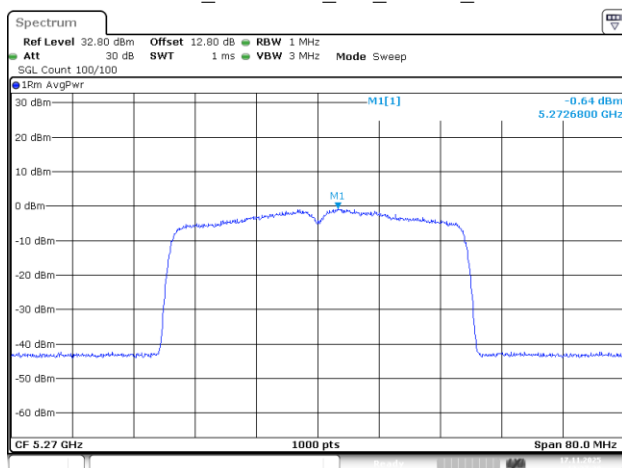
802.11be40_5270MHz_RU_484/65_Chain 3
