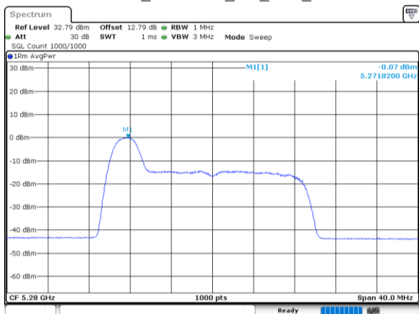
802.11be20_5280MHz_RU_26/0_Chain 3
