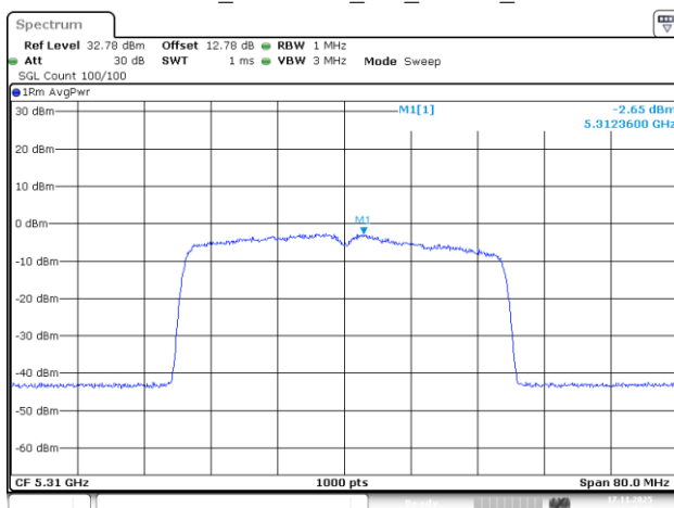
802.11be40_5310MHz_RU_484/65_Chain 3
