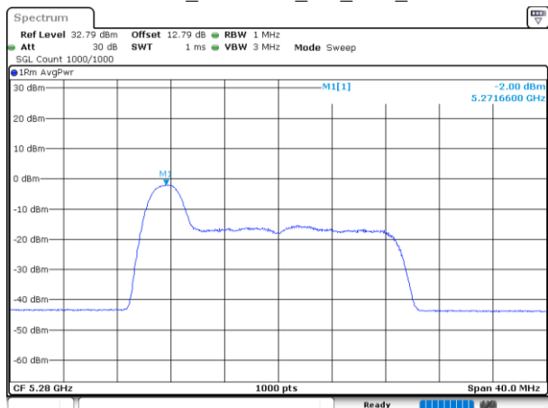
802.11be20_5280MHz_RU_26/0_Chain 1
