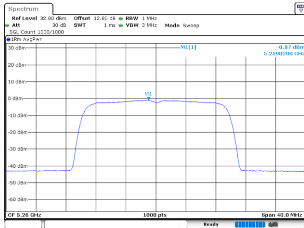
802.11be20_5260MHz_RU_242/61_Chain 2
