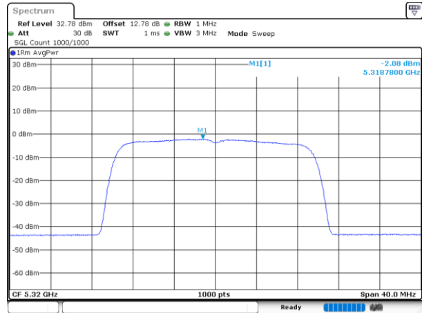
802.11be20_5320MHz_RU_242/61_Chain 1
