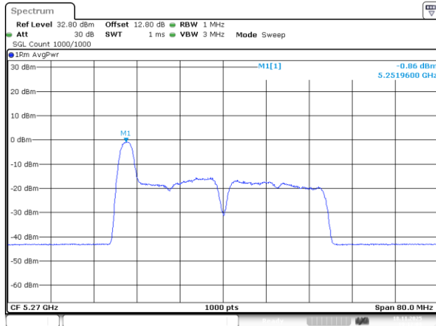
802.11be40_5270MHz_RU_26/0_Chain 0
