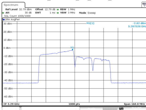
802.11be80_5290MHz_RU_484/65_Chain 2
