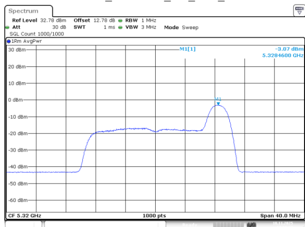
802.11be20_5320MHz_RU_26/8_Chain 3
