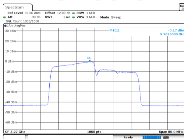
802.11be40_5270MHz_RU_242/61_Chain 3
