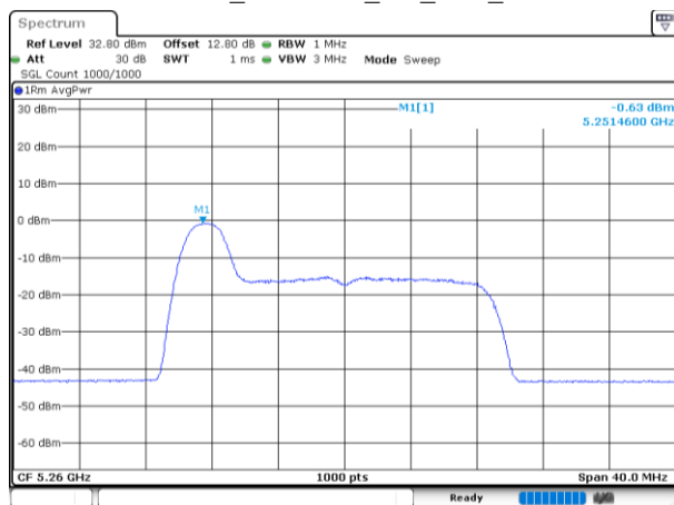
802.11be20_5260MHz_RU_26/0_Chain 2
