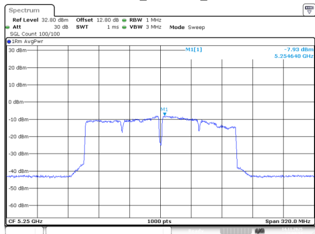
802.11ac160_5250MHz_Chain 3
