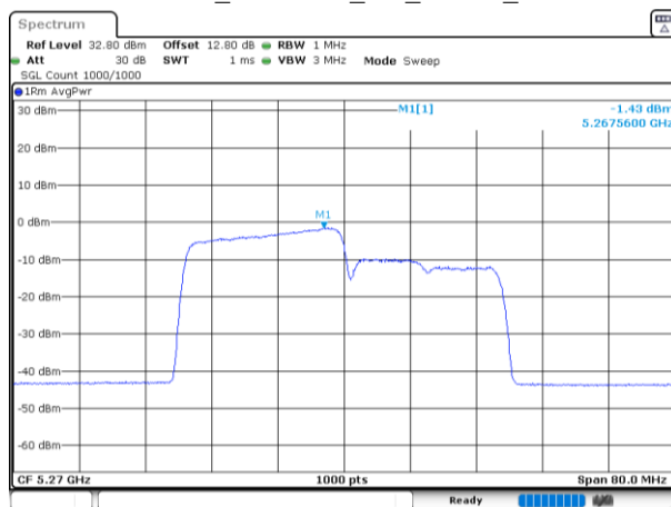
802.11be40_5270MHz_RU_242/61_Chain 0
