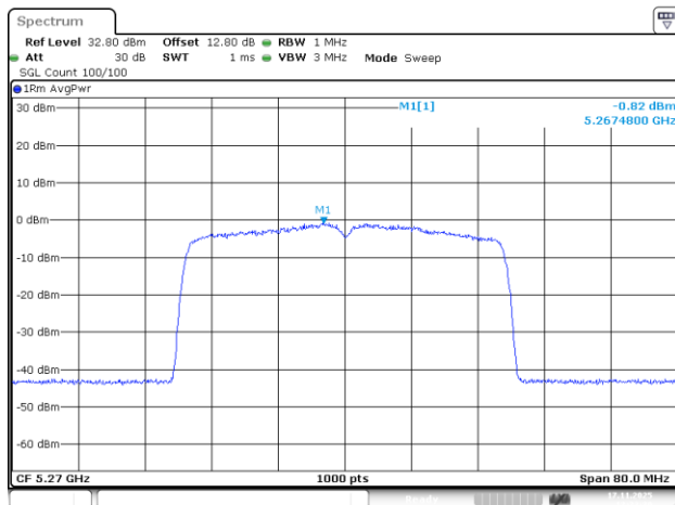
802.11be40_5270MHz_RU_484/65_Chain 0
