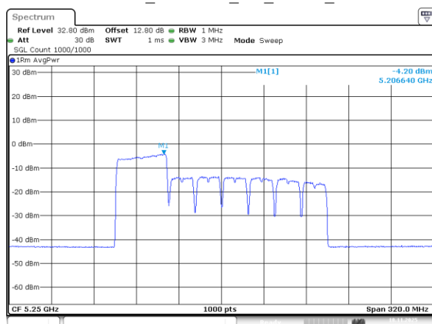
802.11be160_5250MHz_RU_484/65_Chain 2
