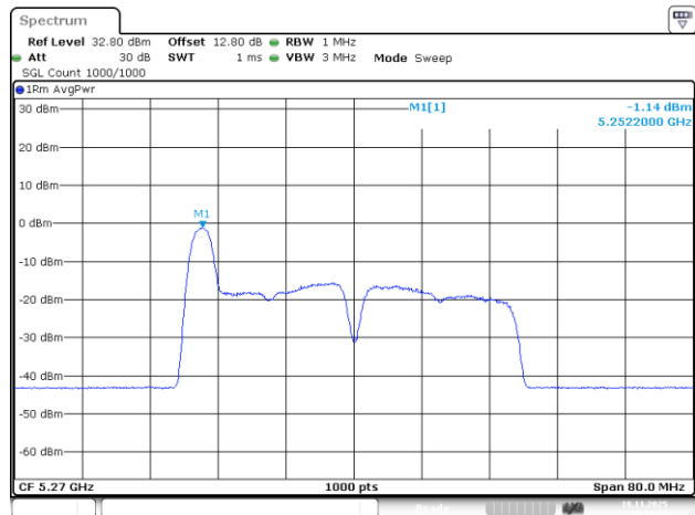
802.11be40_5270MHz_RU_26/0_Chain 3
