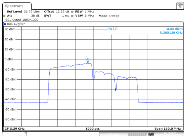
802.11be80_5290MHz_RU_484/65_Chain 3
