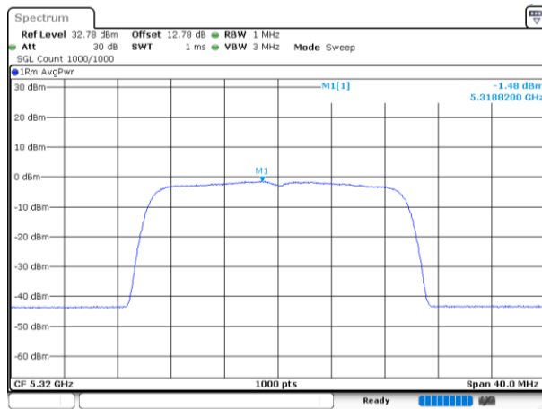
802.11be20_5320MHz_RU_242/61_Chain 0
