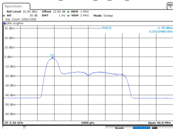
802.11be20_5260MHz_RU_26/0_Chain 1
