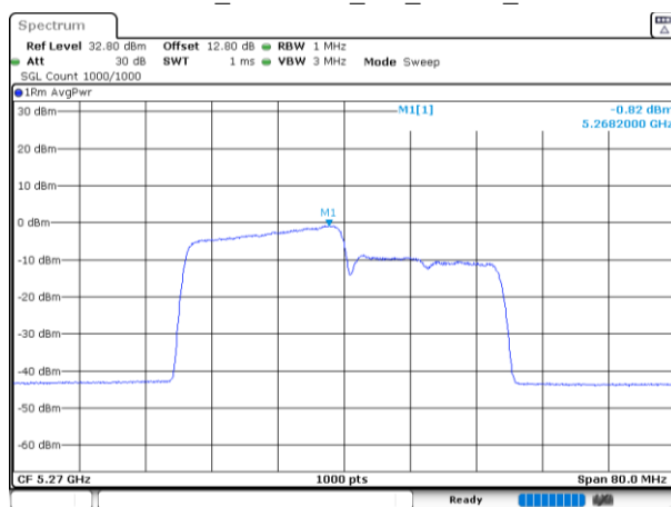
802.11be40_5270MHz_RU_242/61_Chain 2
