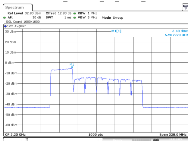
802.11be160_5250MHz_RU_484/65_Chain 0
