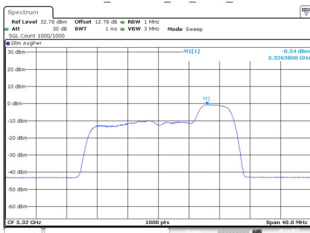
802.11be20_5320MHz_RU_52/40_Chain 2
