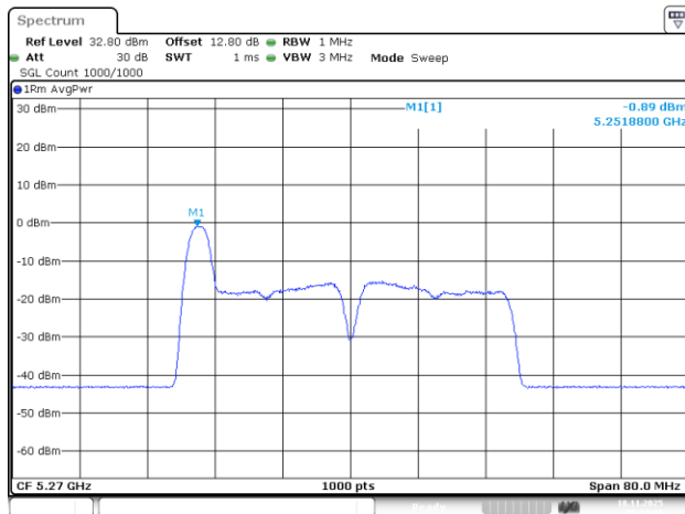
802.11be40_5270MHz_RU_26/0_Chain 2
