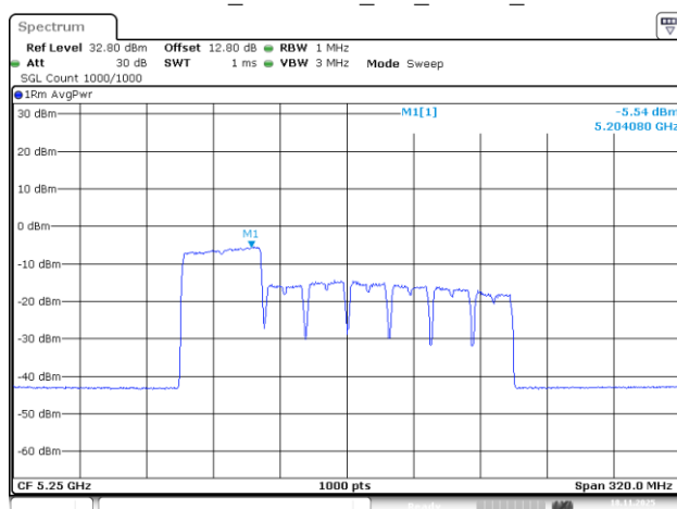
802.11be160_5250MHz_RU_484/65_Chain 1
