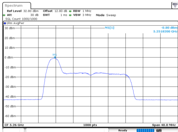
802.11be20_5260MHz_RU_26/0_Chain 0
