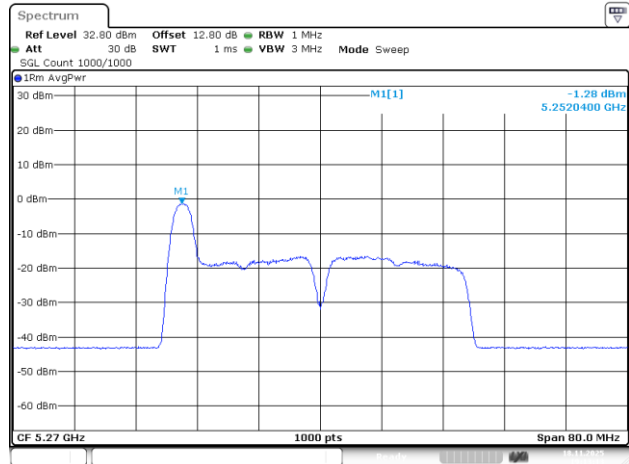
802.11be40_5270MHz_RU_26/0_Chain 1
