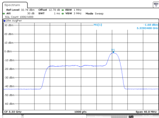
802.11be20_5320MHz_RU_26/8_Chain 1
