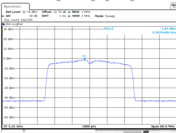
802.11be40_5310MHz_RU_484/65_Chain 1
