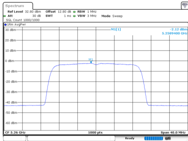
802.11be20_5260MHz_RU_242/61_Chain 1
