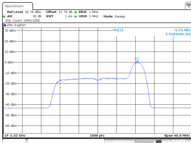
802.11be20_5320MHz_RU_26/8_Chain 0
