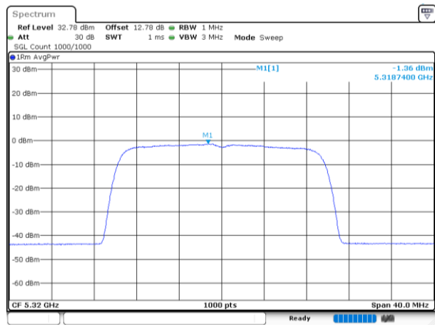
802.11be20_5320MHz_RU_242/61_Chain 3
