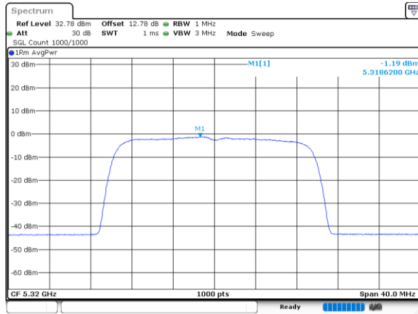
802.11be20_5320MHz_RU_242/61_Chain 2
