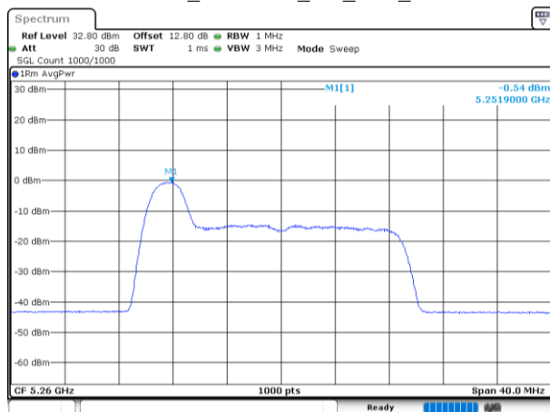
802.11be20_5260MHz_RU_26/0_Chain 3
