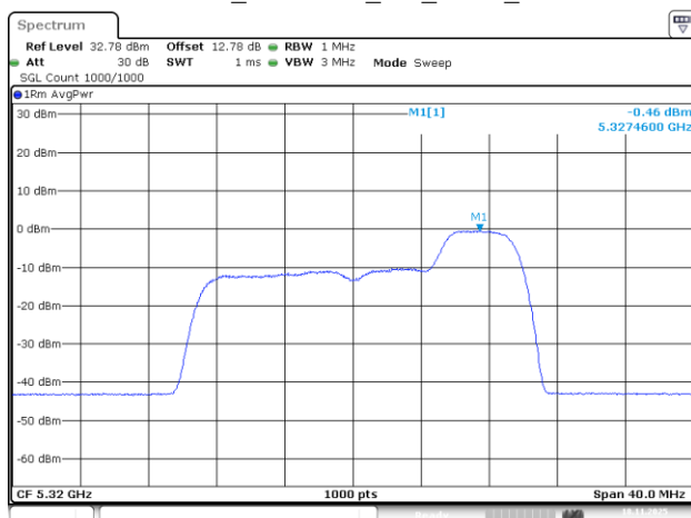
802.11be20_5320MHz_RU_52/40_Chain 0
