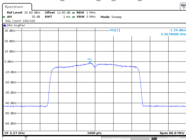
802.11be40_5270MHz_RU_484/65_Chain 1
