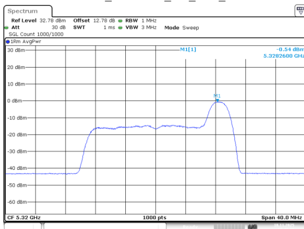
802.11be20_5320MHz_RU_26/8_Chain 2
