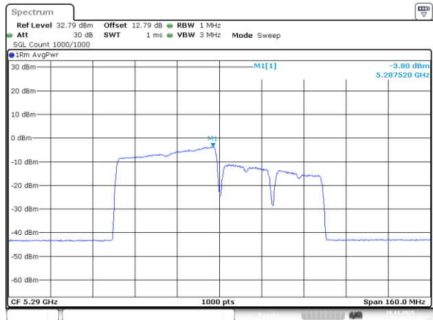
802.11be80_5290MHz_RU_484/65_Chain 1
