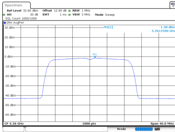
802.11be20_5260MHz_RU_242/61_Chain 0
