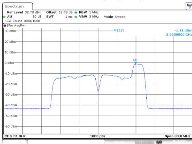
802.11be40_5310MHz_RU_52/44_Chain 2
