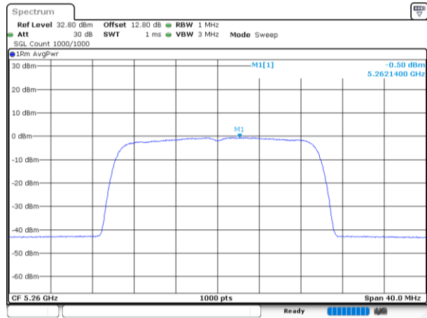
802.11be20_5260MHz_RU_242/61_Chain 3
