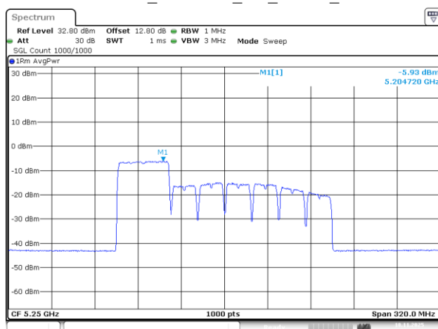
802.11be160_5250MHz_RU_484/65_Chain 3
