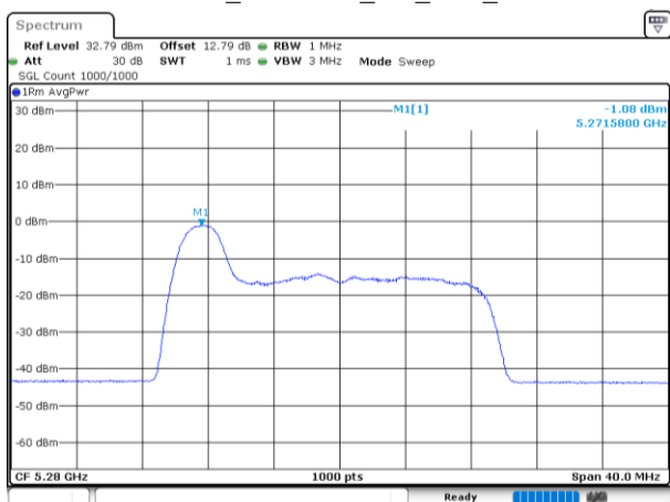
802.11be20_5280MHz_RU_26/0_Chain 2
