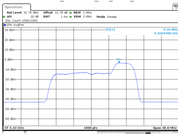
802.11be20_5320MHz_RU_52/40_Chain 3
