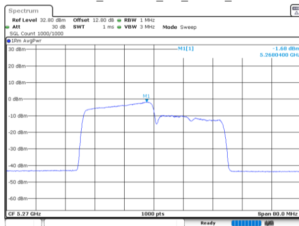
802.11be40_5270MHz_RU_242/61_Chain 1
