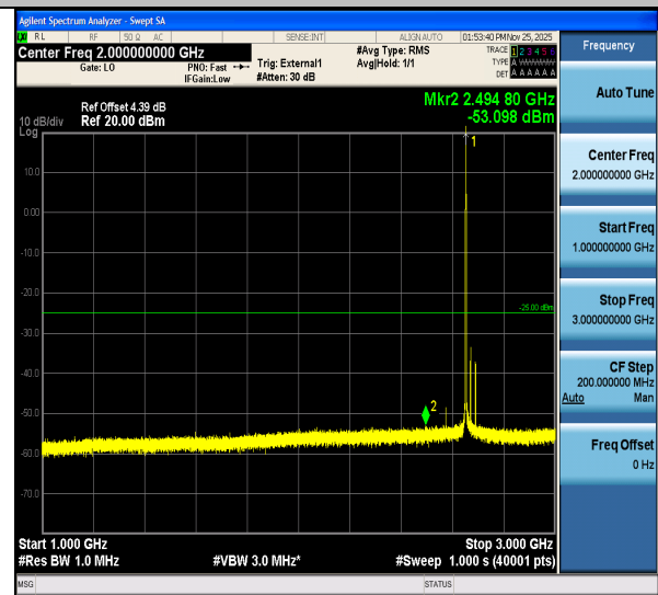
CA_41C-20MHz-20MHz-QPSK-QPSK-41292-41490-1RB#0- ORB#0-1000~3000MHz-PASS
