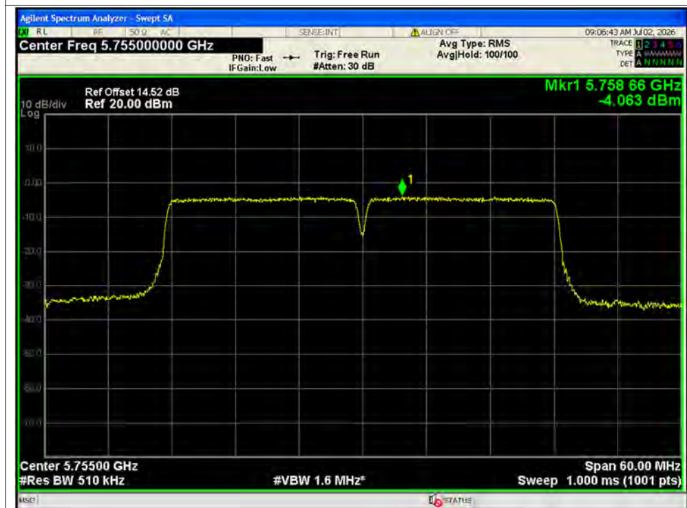
PSD NVNT n40 5755MHz Ant2 MIMO
