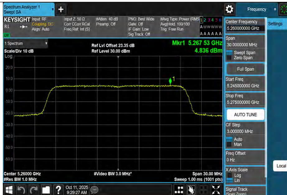
11AX20MIMO-Ant1-5260-PASS
