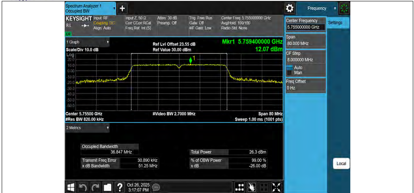
11AC40MIMO-Ant1-5755
