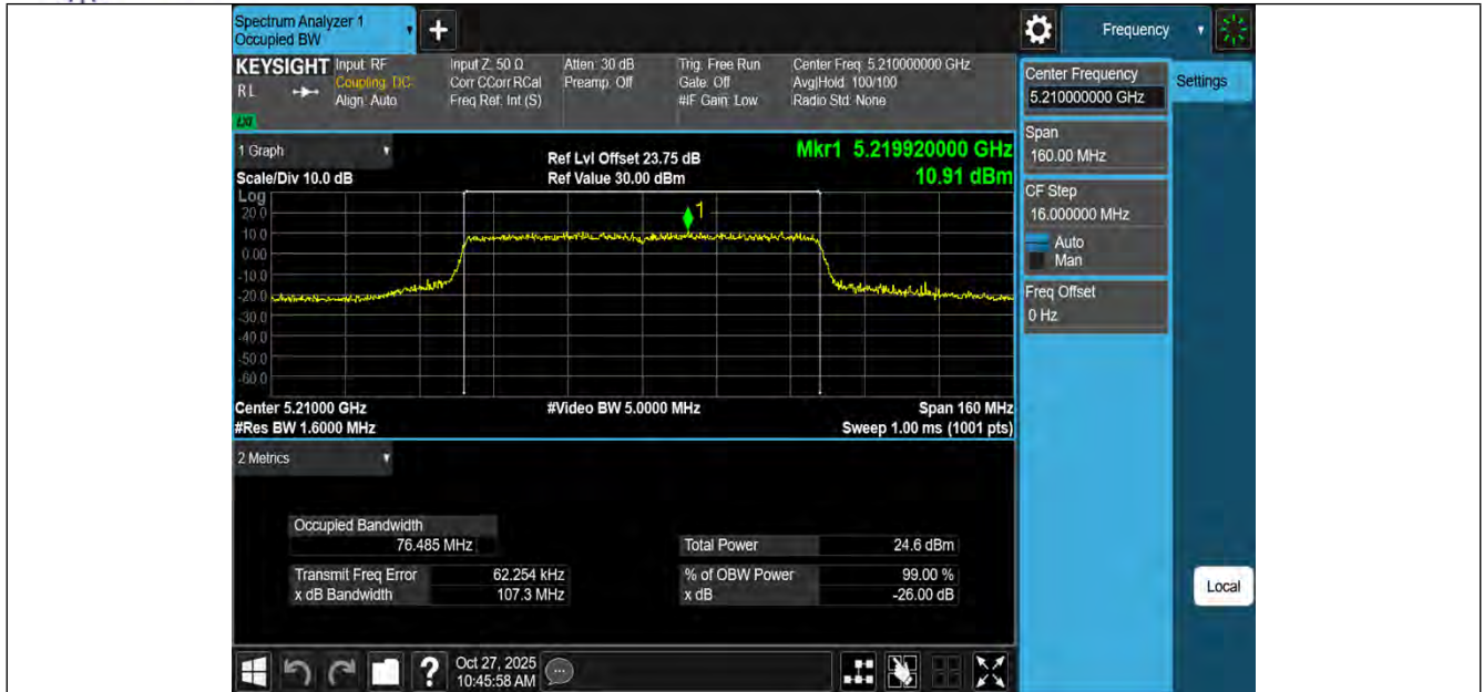
11AC80MIMO-Ant1-5210
