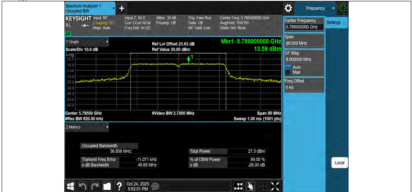
11N40MIMO-Ant1-5795
