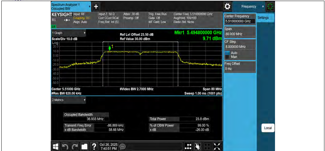
11N40MIMO-Ant1-5510
