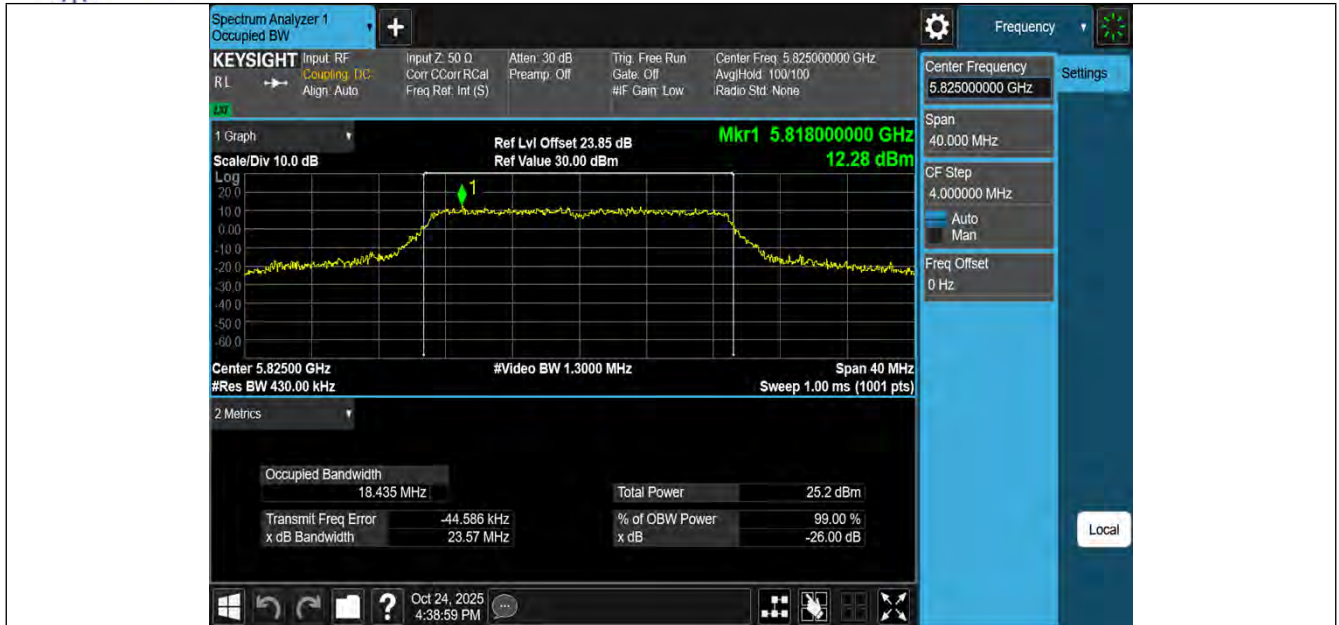
11N20MIMO-Ant3-5825
