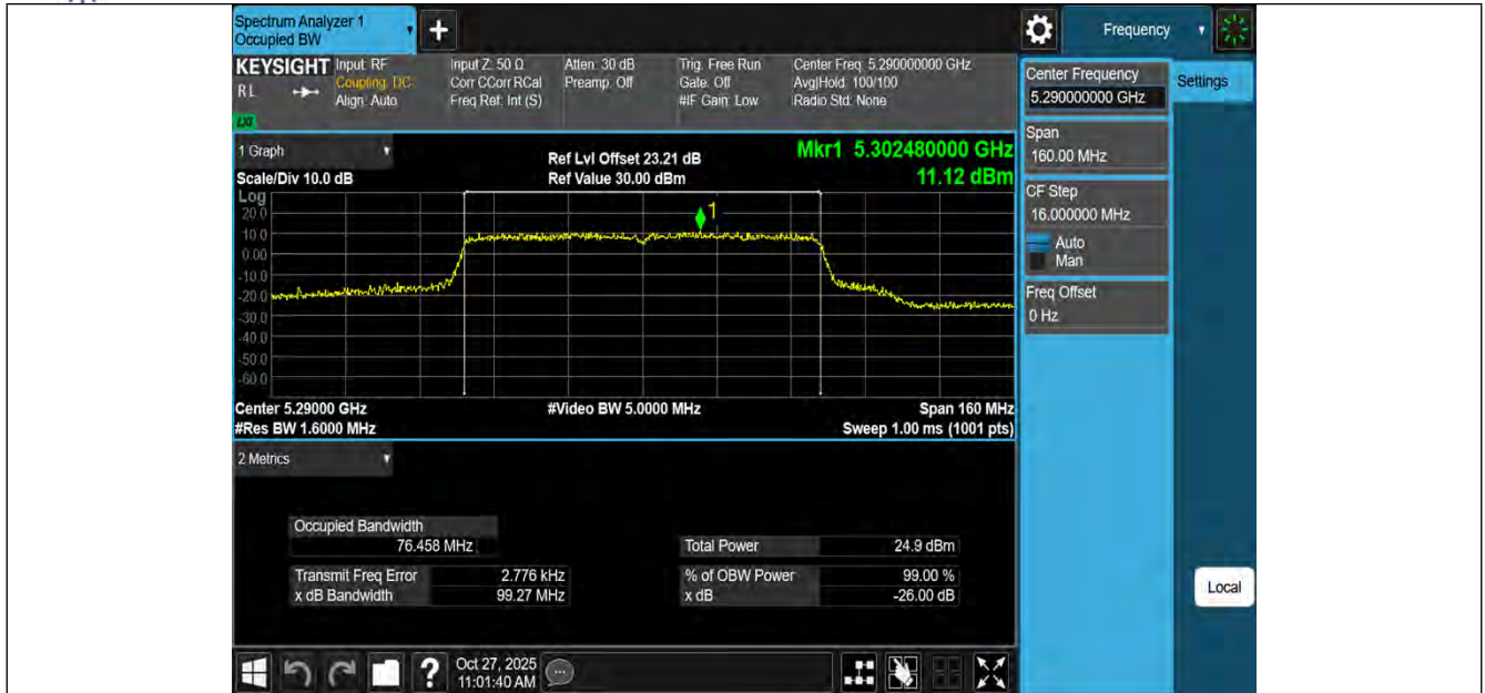
11AC80MIMO-Ant1-5290
