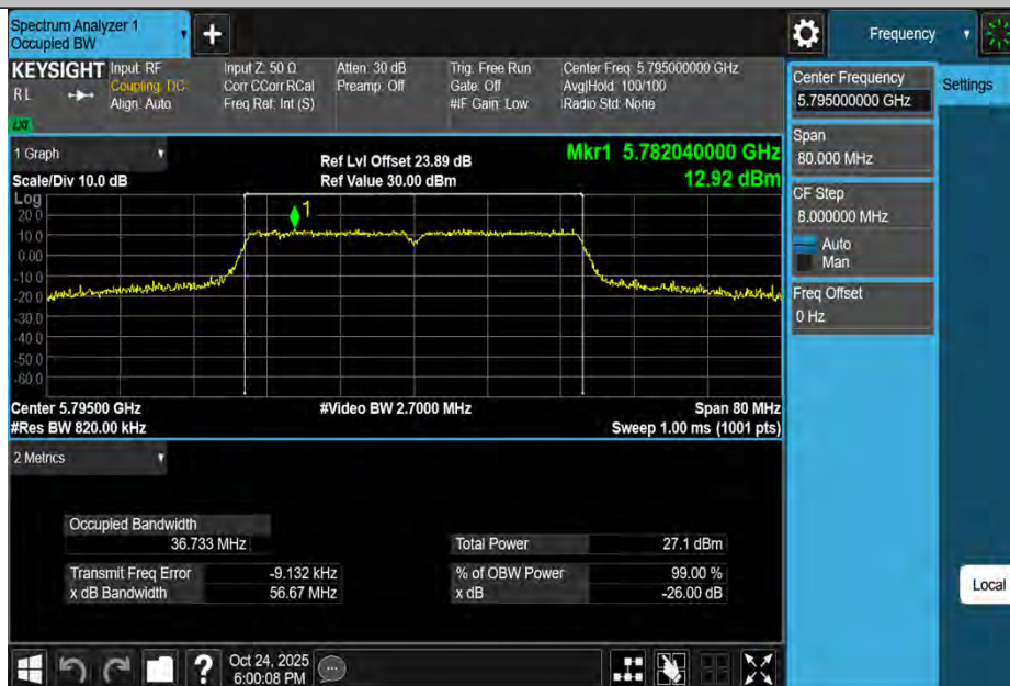
11N40MIMO-Ant4-5795
