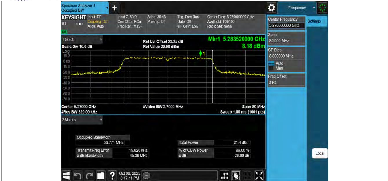
11N40MIMO-Ant3-5270
