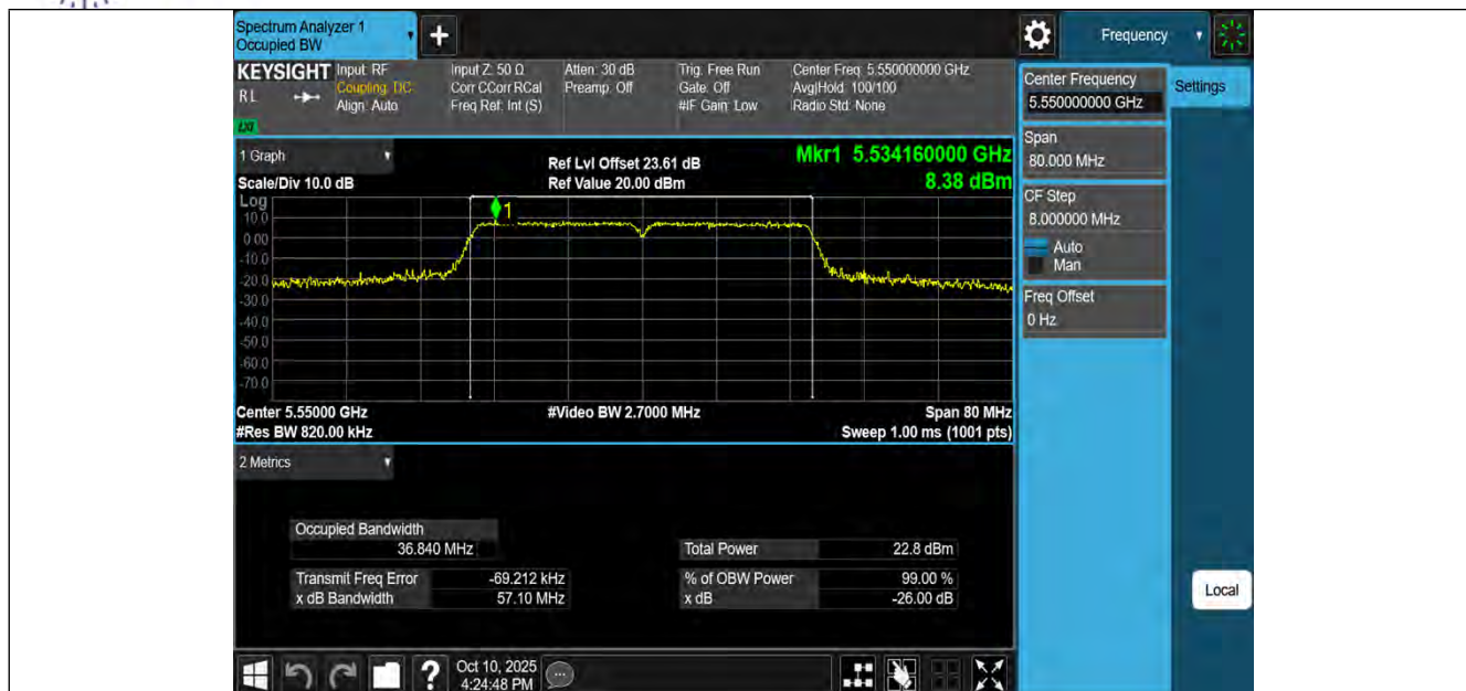
11AC40MIMO-Ant1-5550
