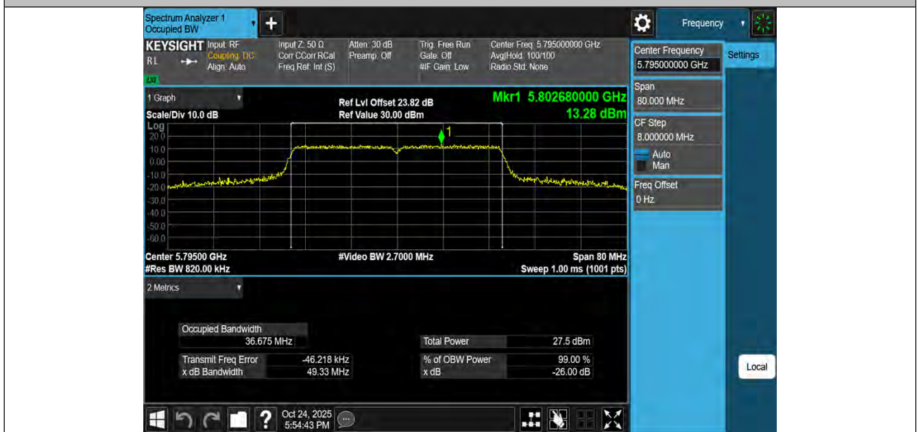
11N40MIMO-Ant2-5795
