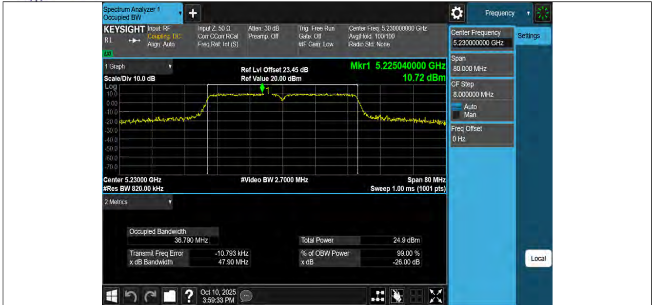
11AC40MIMO-Ant1-5230
