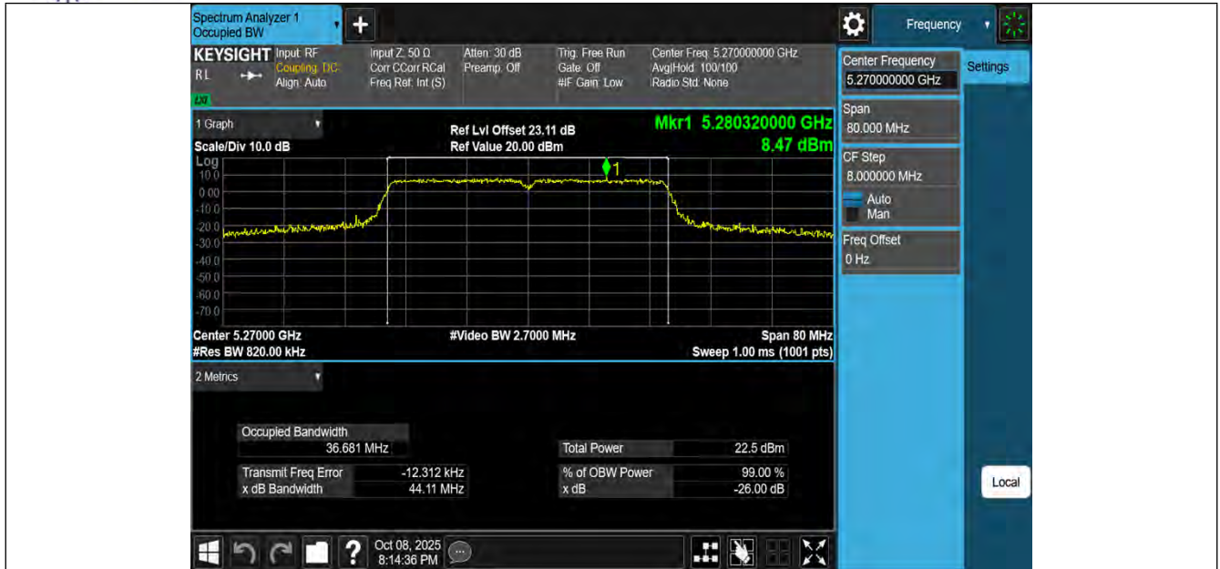
11N40MIMO-Ant1-5270
