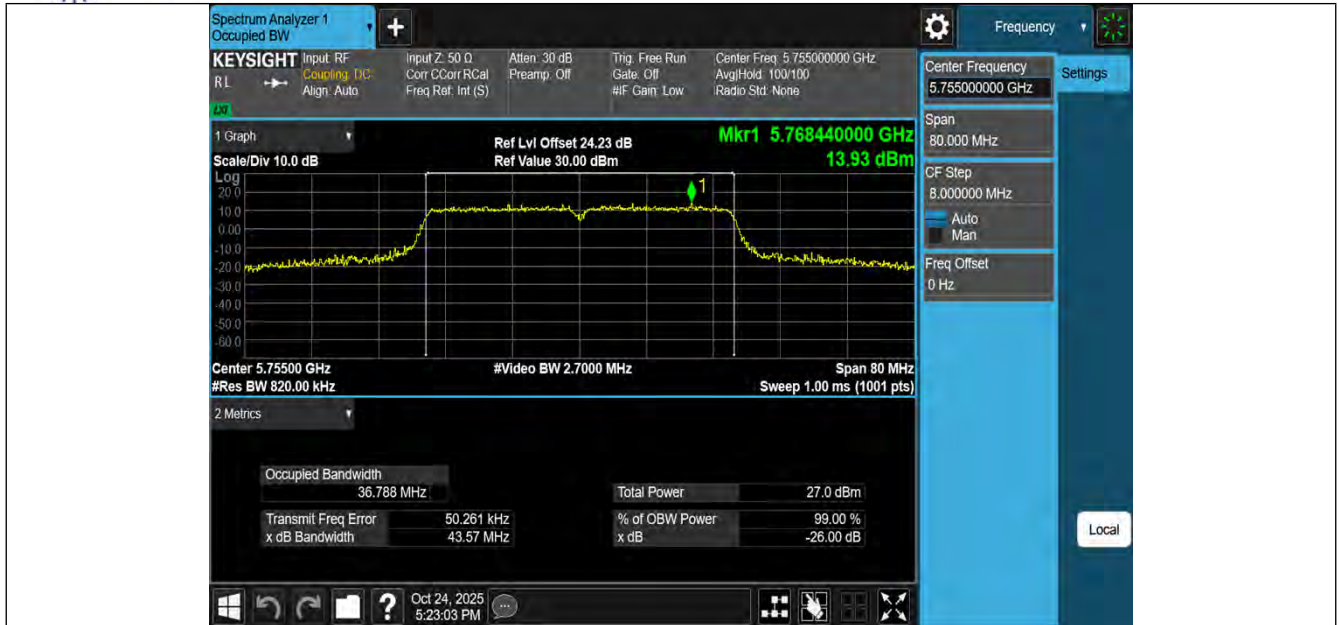
11N40MIMO-Ant3-5755
