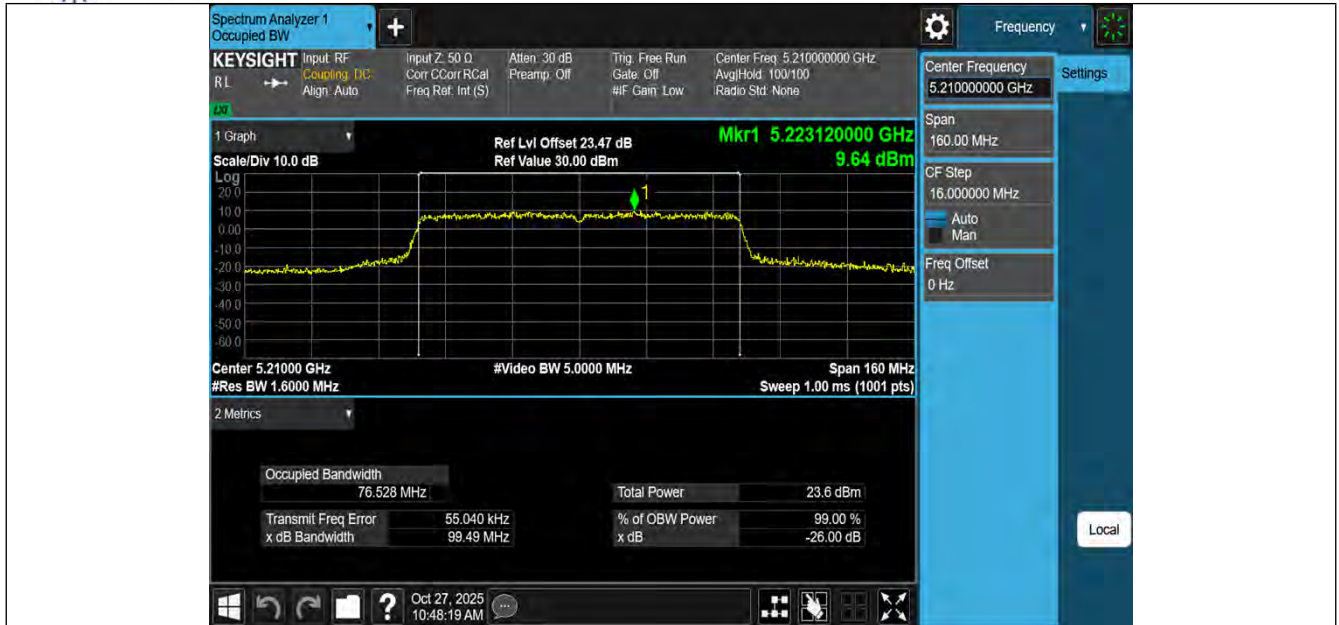
11AC80MIMO-Ant3-5210
