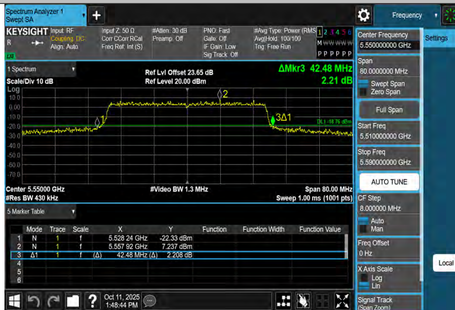
11AX40MIMO-Ant3-5550
