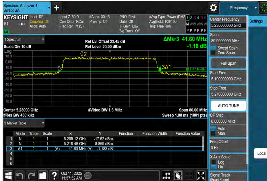
11AX40MIMO-Ant1-5230
