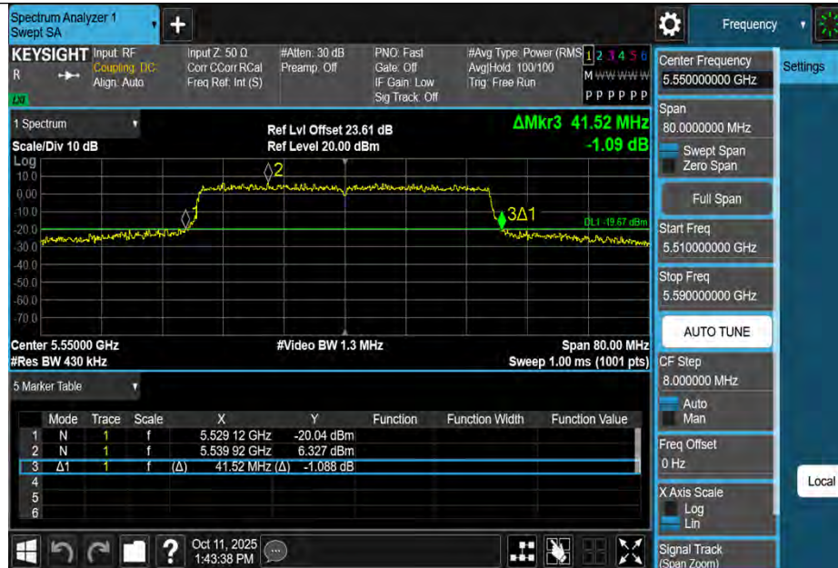
11AX40MIMO-Ant1-5550
