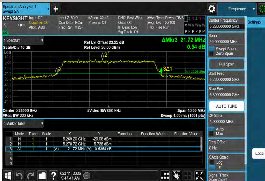
11AX20MIMO-Ant3-5280
