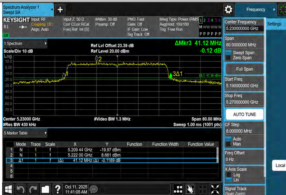
11AX40MIMO-Ant4-5230
