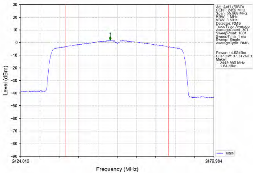
802.11ax(HE40) HCH 2452MHz SU / Ant1 (SISO) NTNV
