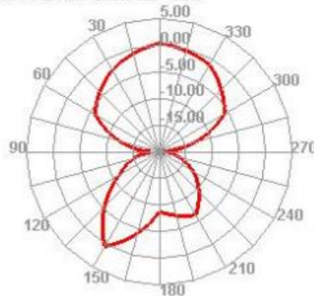
2450.000MHz E2
