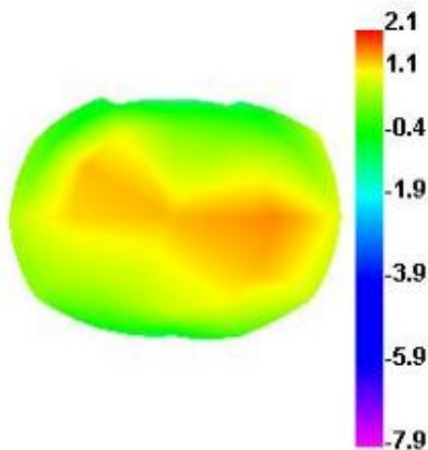
2450.000MHz E1
