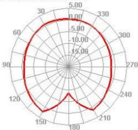
2450.000MHz E1
