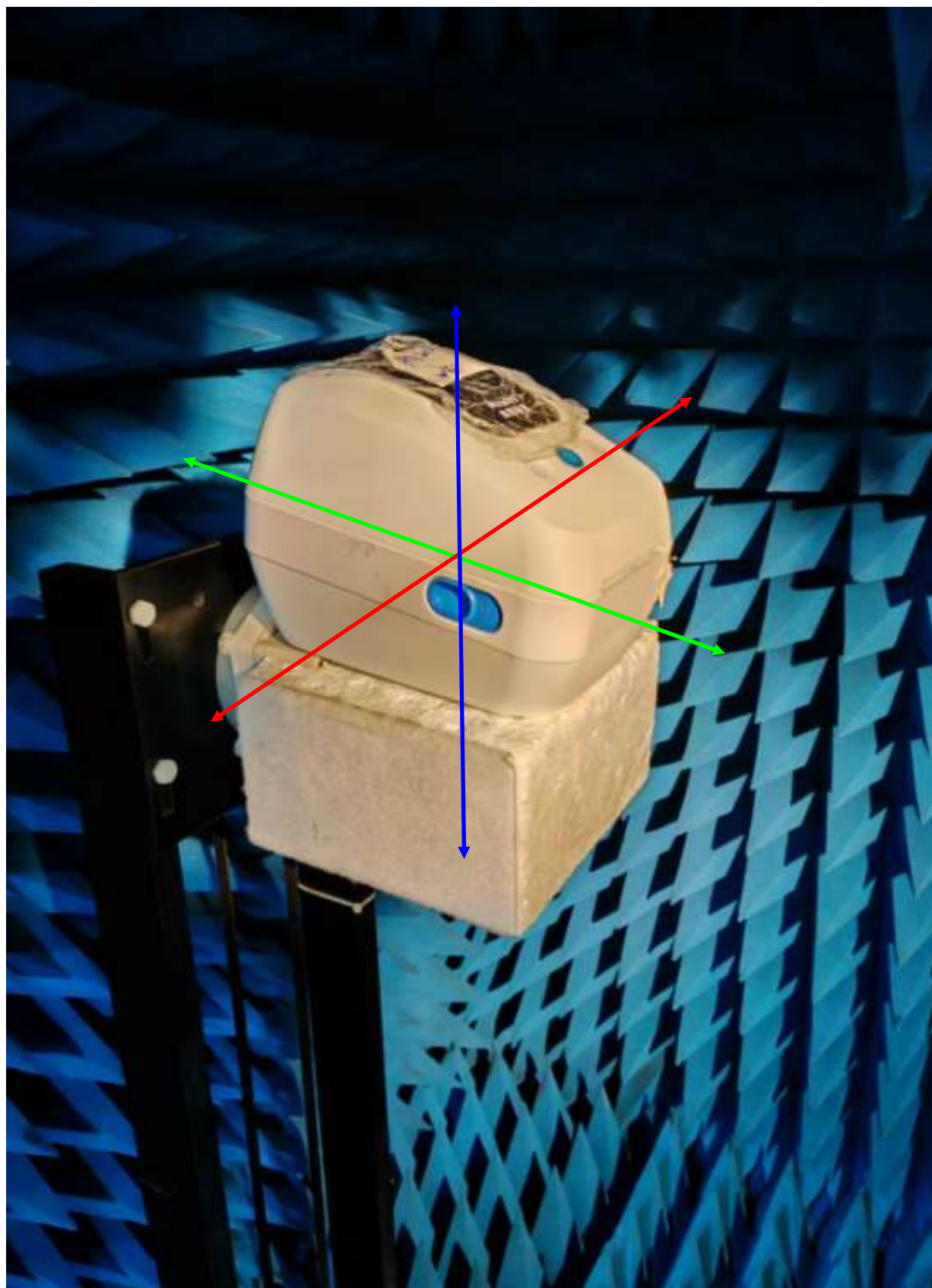
OTA 暗室图
