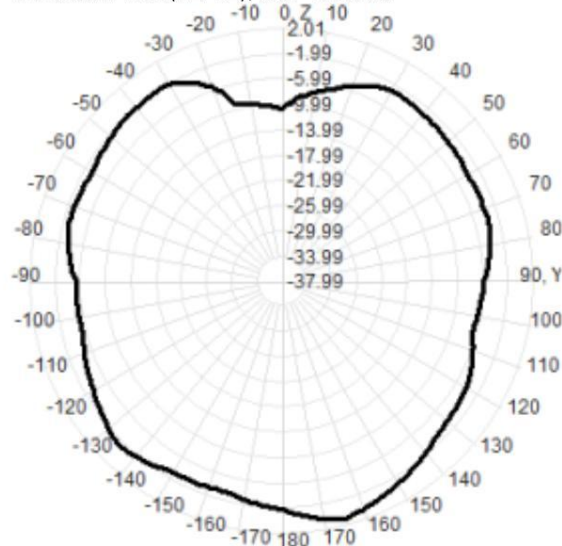
1770.0MHz Total(E2-YZ), Max= 0.65dBi
