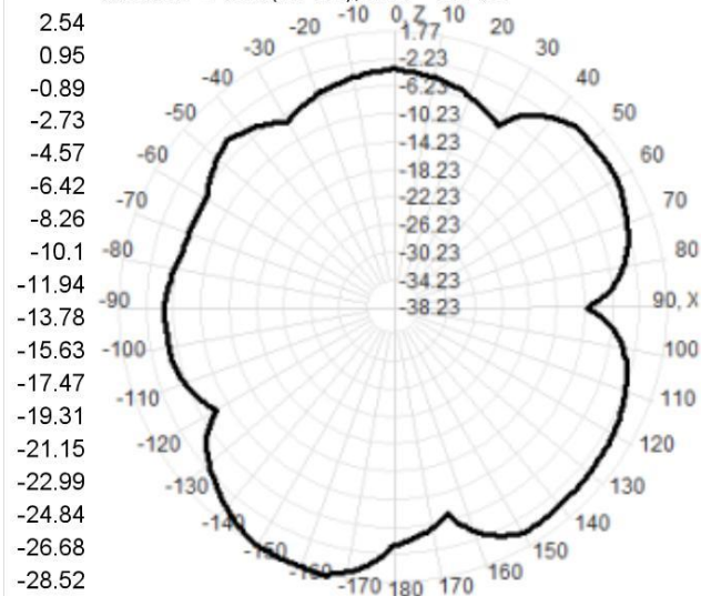
1850.0MHz Total(E1-XZ), Max= 1.77dBi
