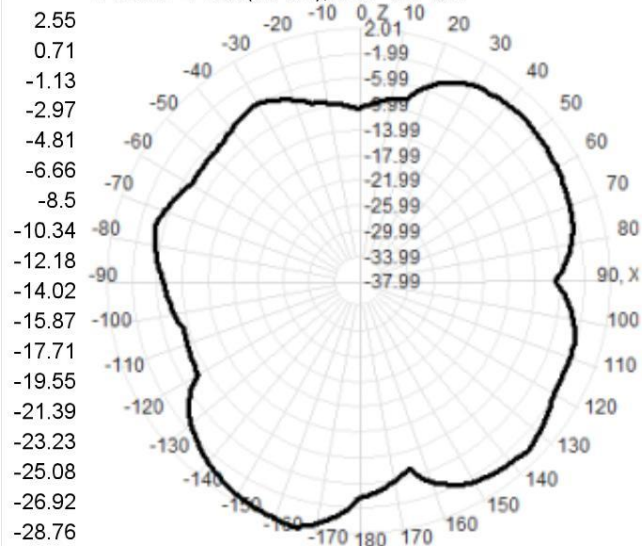
1770.0MHz Total(E1-XZ), Max= 2.01dBi
