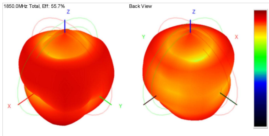
1850.0MHz Total(E1-XZ), Max= 1.77dBi
