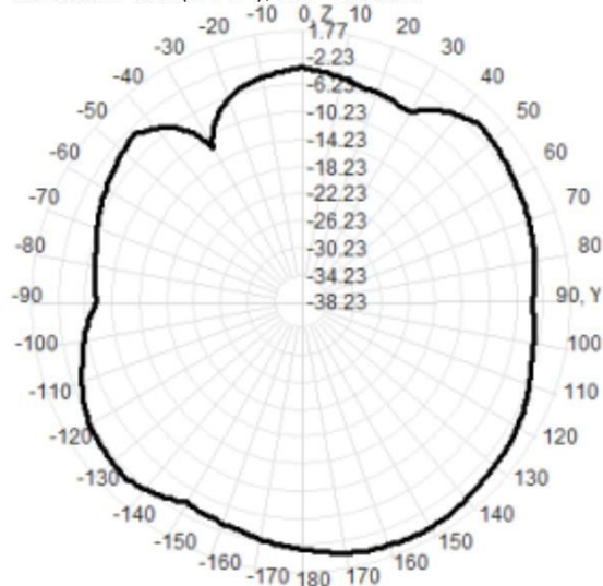
1850.0MHz Total(E2-YZ), Max= 0.07dBi
