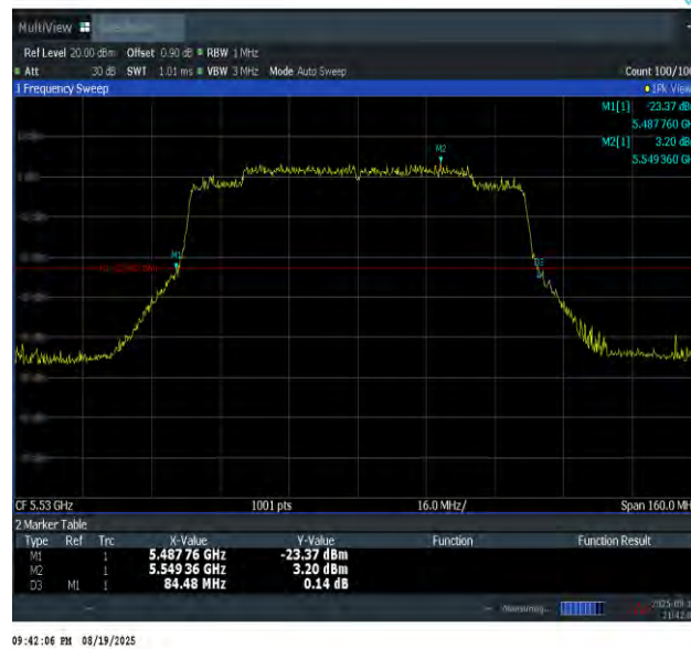
11AX80SISO-Ant1-5530
