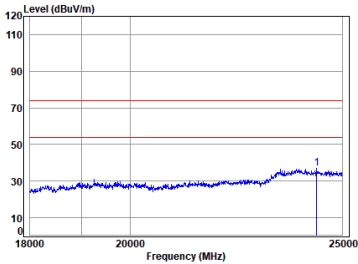
BLE 1M_TX_CH_M_Horizontal
