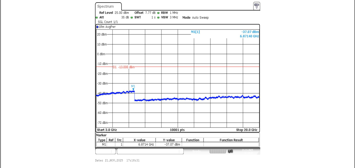
Band4-1312-1-3000~20000MHz-PASS
