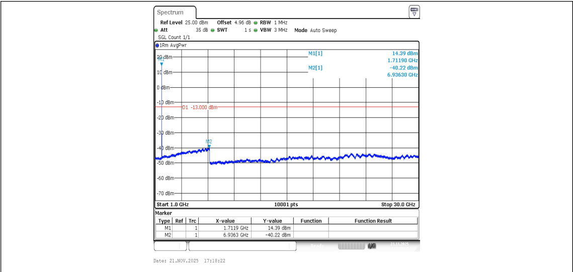
Band4-1312-1-1000~30000MHz-PASS
