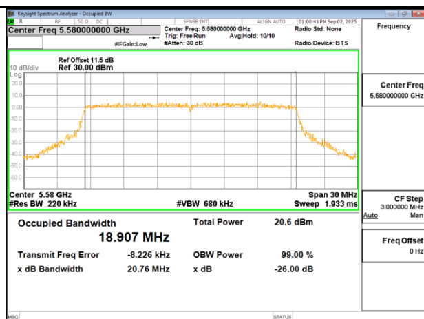
802.11ax 20MHz Chain1 5580MHz
