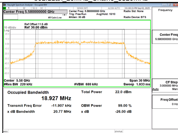
802.11ax 20MHz Chain0 5580MHz
