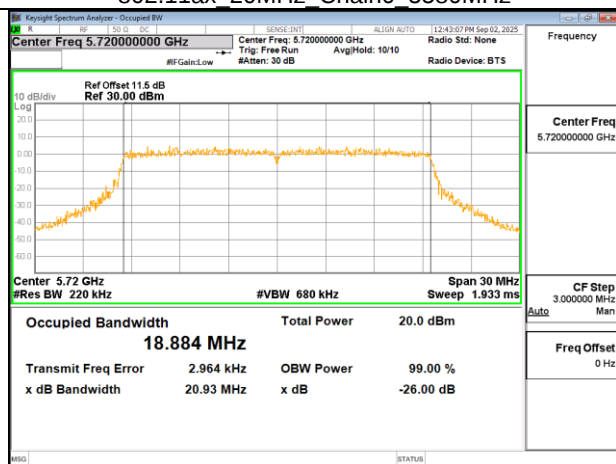
802.11ax 20MHz Chain0 5720MHz
