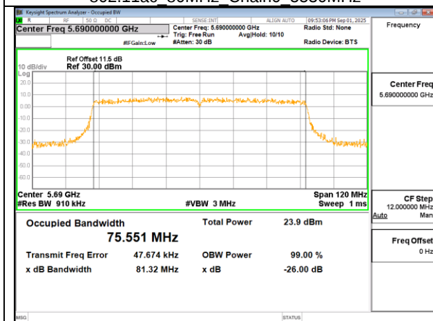
802.11ac 80MHz Chain0 5690MHz
