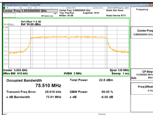
802.11ac 80MHz Chain1 5855MHz
