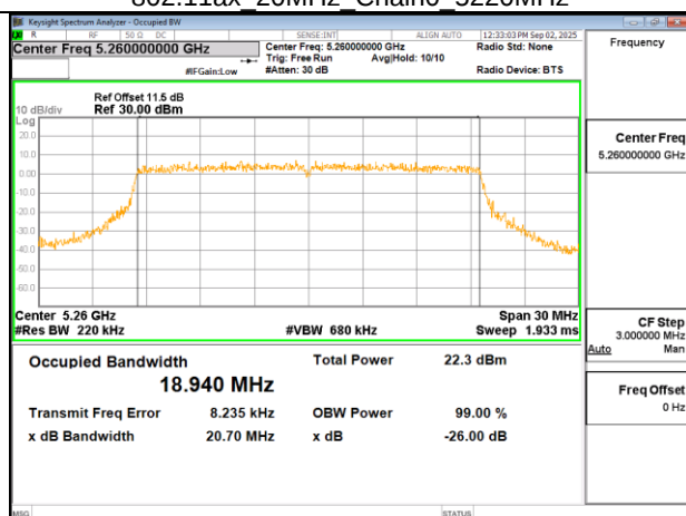
802.11ax 20MHz Chain0 5260MHz
