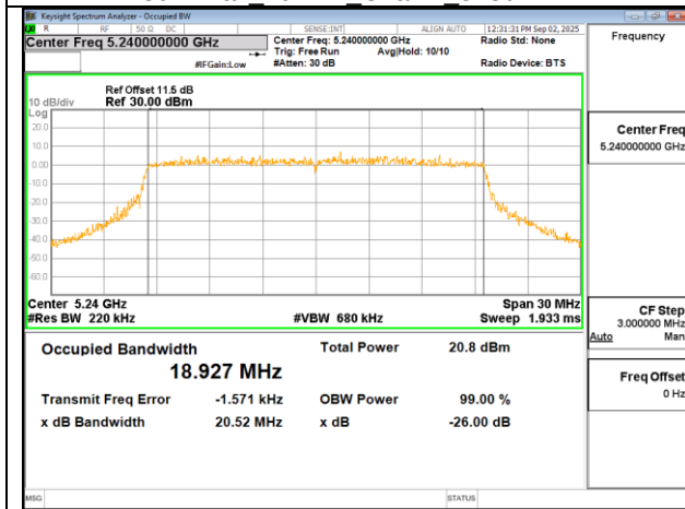
802.11ax 20MHz Chain1 5240MHz
