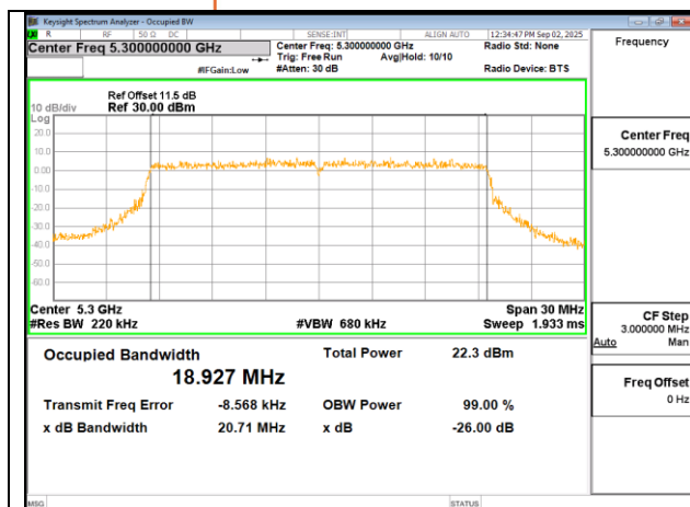
802.11ax 20MHz Chain0 5300MHz
