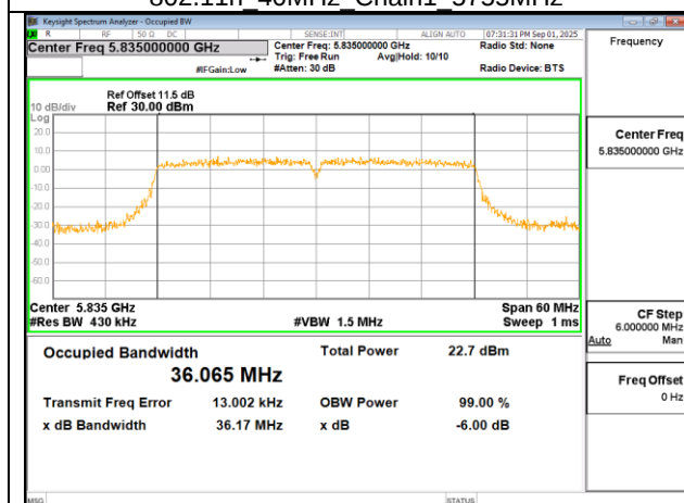
802.11n 40MHz Chain1 5835MHz
