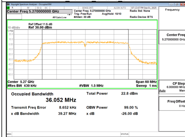
802.11n 40MHz Chain0 5270MHz
