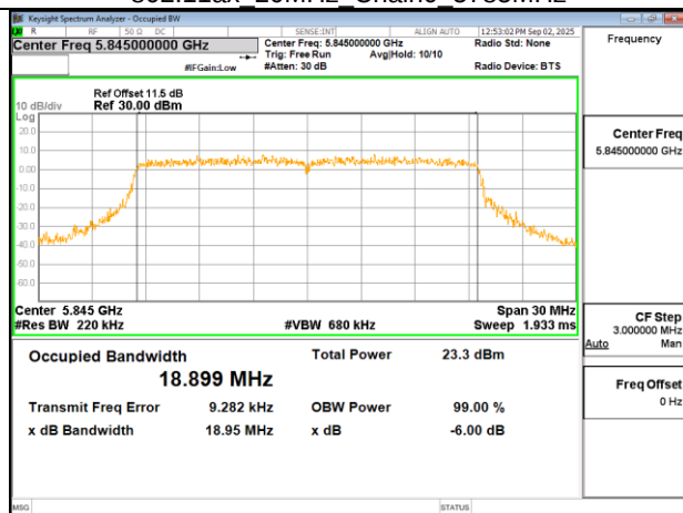
802.11ax 20MHz Chain0 5845MHz
