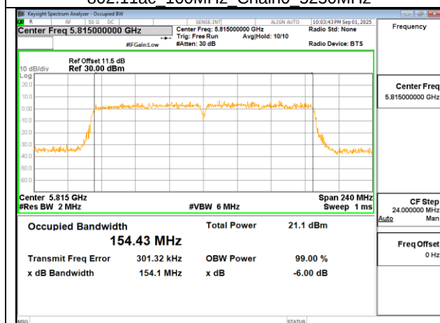
802.11ac 160MHz Chain0 5815MHz
