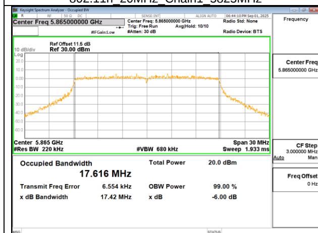
802.11n 20MHz Chain1 5865MHz
