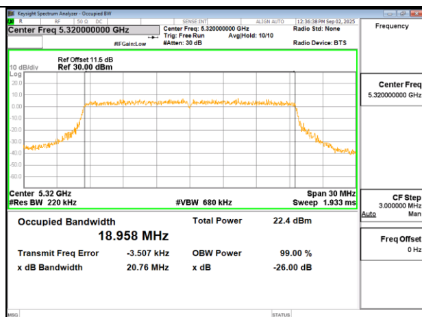
802.11ax 20MHz Chain0 5320MHz
