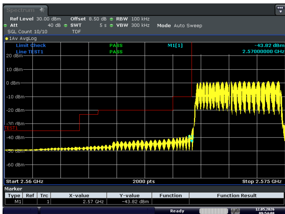
Test_Graph_band38_2572.5MHz_5M_QPSK_1RB#LOW_Band edge
