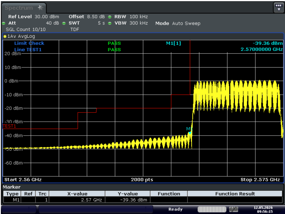
Test_Graph_band38_2572.5MHz_5M_16QAM_1RB#LOW_Band edge
