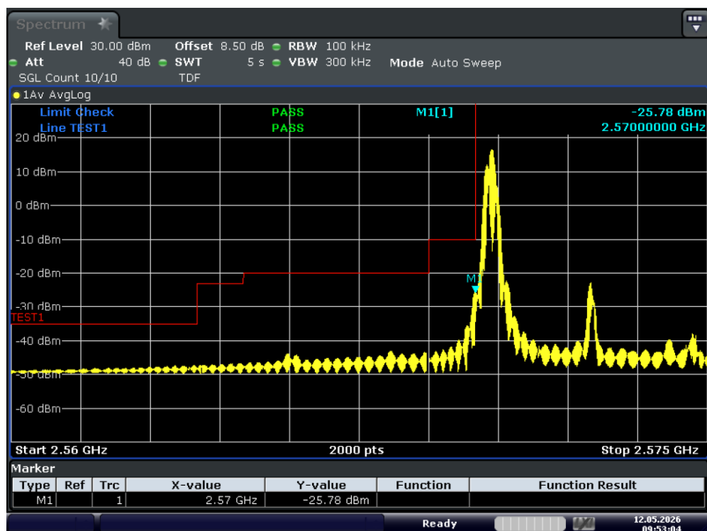
Test_Graph_band38_2572.5MHz_5M_QPSK_1RB#LOW_Band edge
