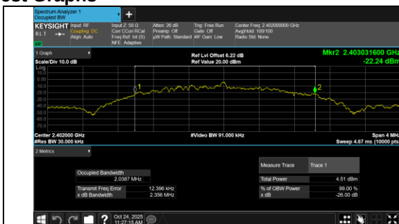
BLE 2M Channel 0
