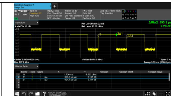
BLE 1M_Channel 19
