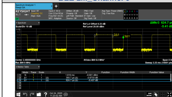
BLE 1M_Channel 39
