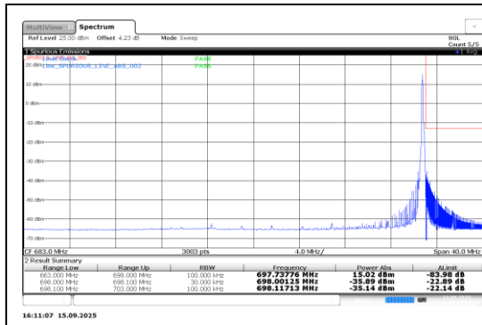
Band71-0.18-BPSK-133470-1@0-15kHz-PASS
