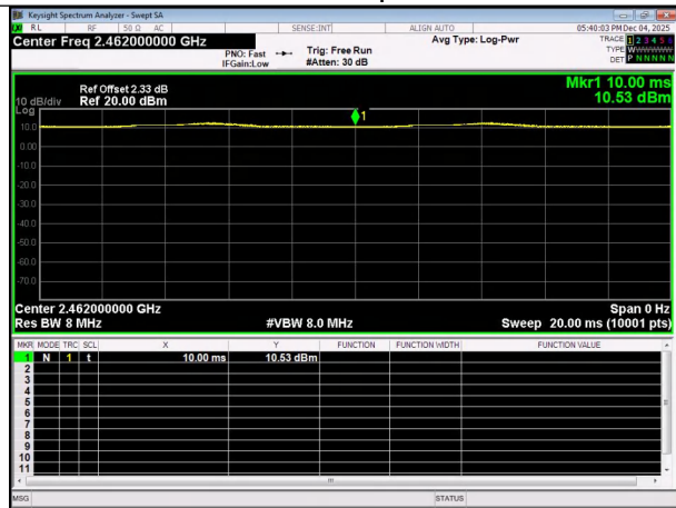
802.11b 1Mbps 2462
