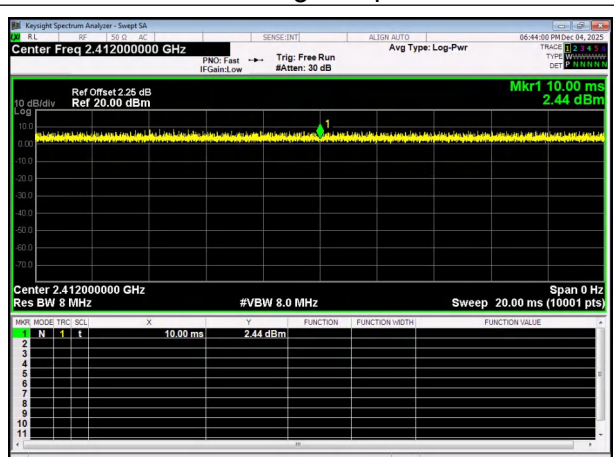
802.11g 6Mbps 2412
