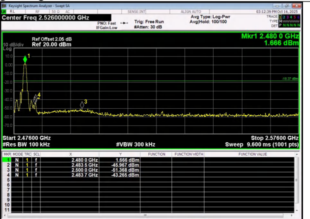
BLE 1M: Band Edge, Right Side
