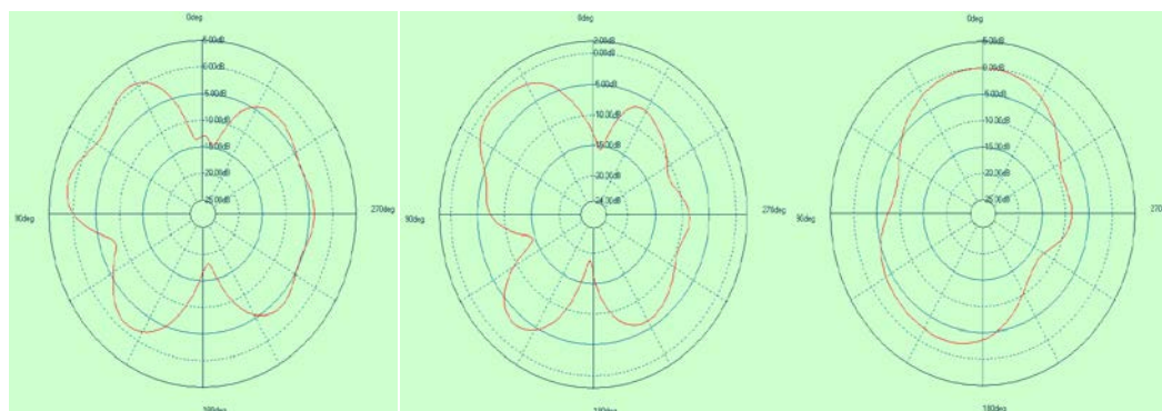
2610MHz (Phi0/Phi90/Theta90)
