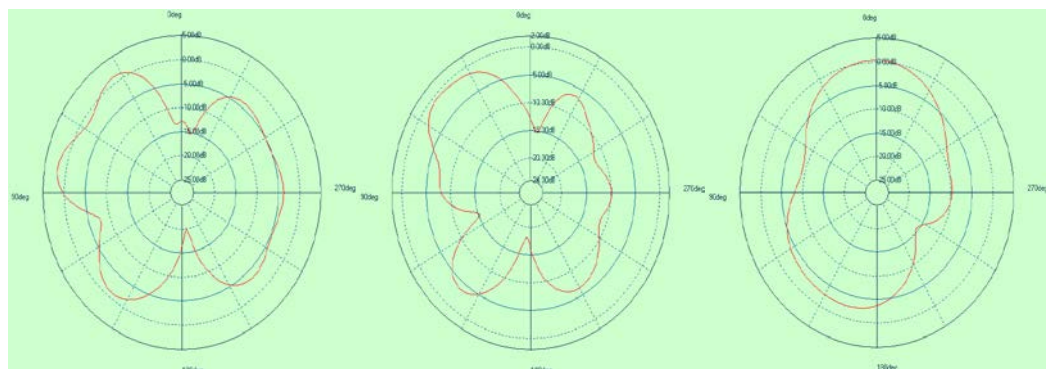
2610MHz (Phi0/Phi90/Theta90)
