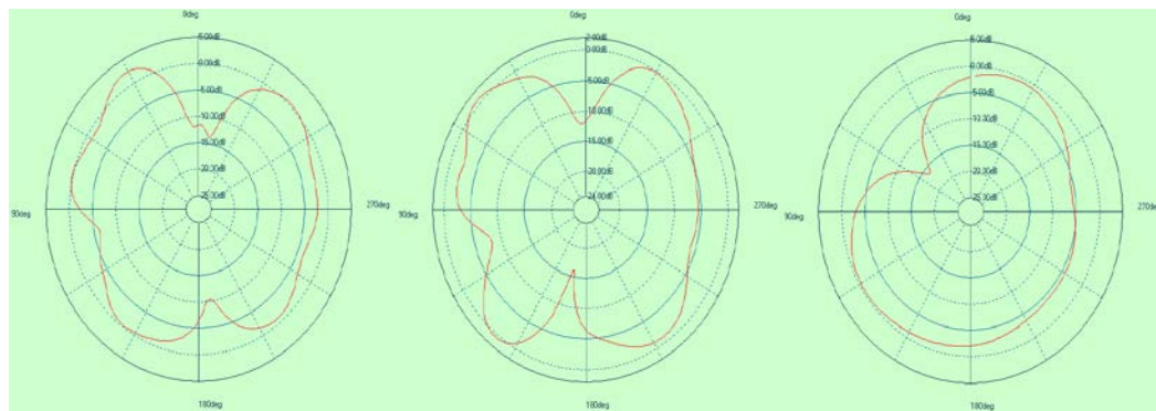
2150MHz (Phi0/Phi90/Theta90)
