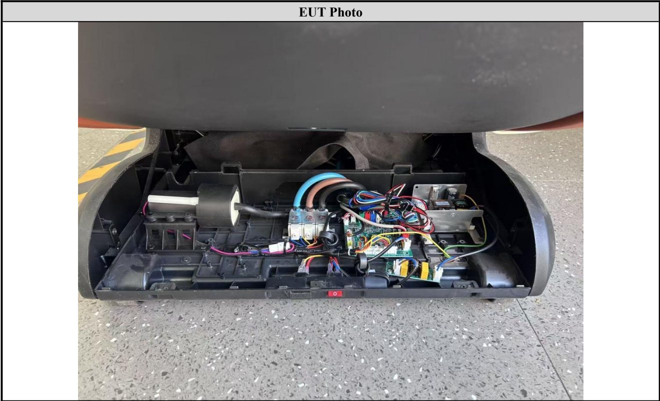
EUT Photo
