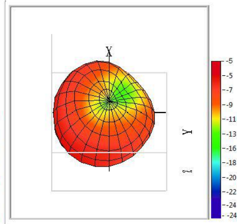
2.485GHzDo
