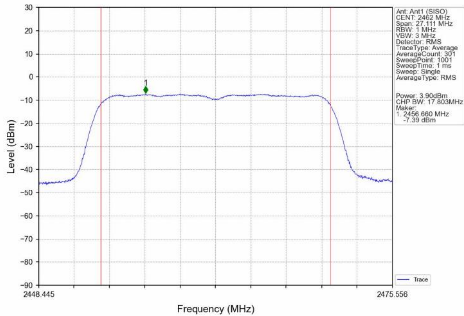
802.11n(HT20) HCH 2462MHz Ant1 (SISO) NTVN
