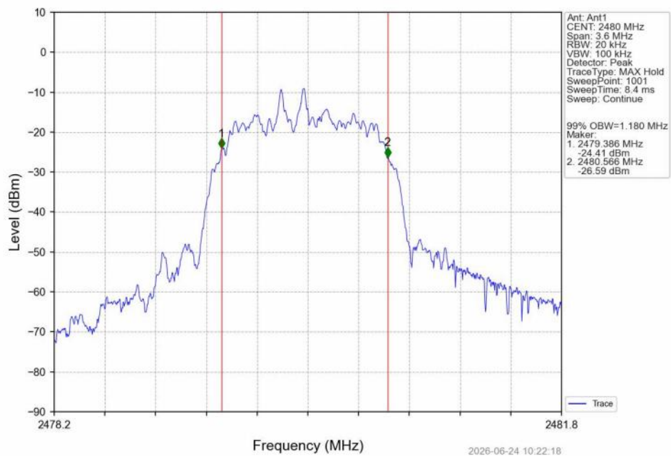
Pi/4DQPSK_2DH5_HCH_2480MHz_Left_NTNV
