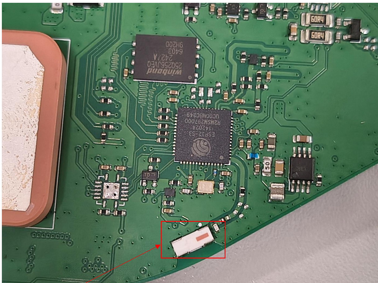
BLE antenna
