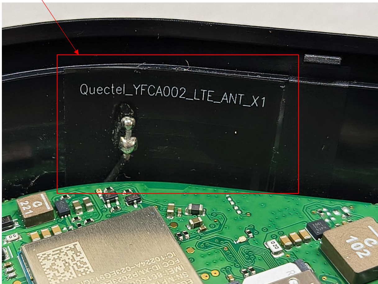
LTE antenna
