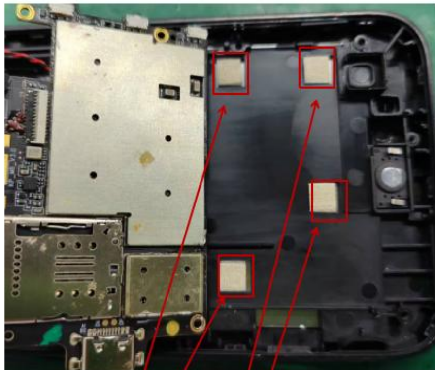
屏上贴导电泡棉与主板接地
