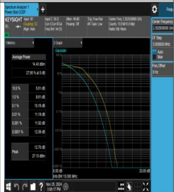
40(2345-2360)-10MHz-16QAM-39175-50RB#0-PA
