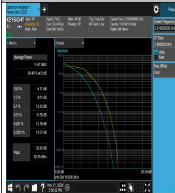
40(2305-2320)-10MHz-QPSK-38750-50RB#0-PA
