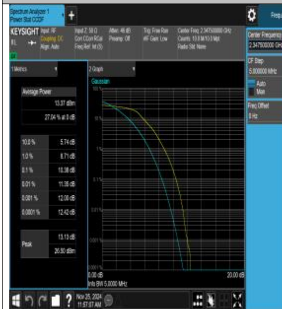
40(2345-2360)-5MHz-QPSK-39125-25RB#0-PAS
