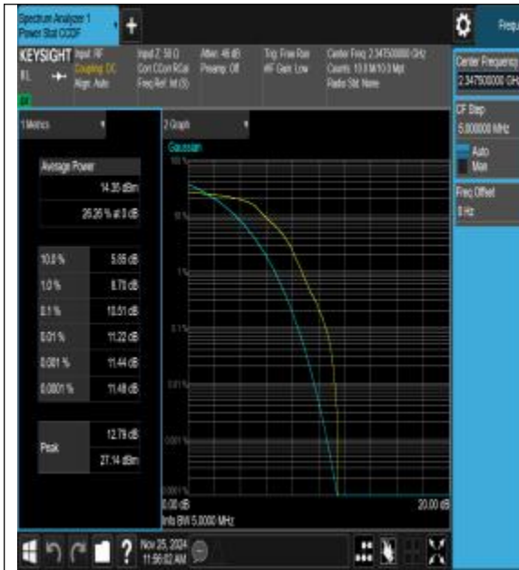
40(2345-2360)-5MHz-QPSK-39125-1RB#0-PASS
