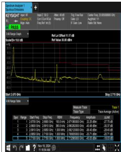
Band41_20MHz_QPSK_41490_1RB#0
