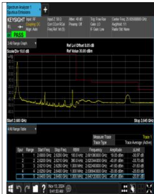
Band38_20MHz_QPSK_38150_1RB#0
