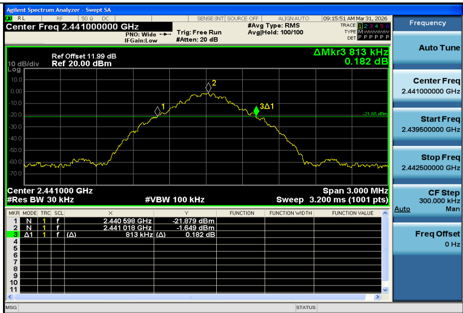
DH5-Ant1-2441
