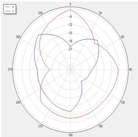
2480 Polar
