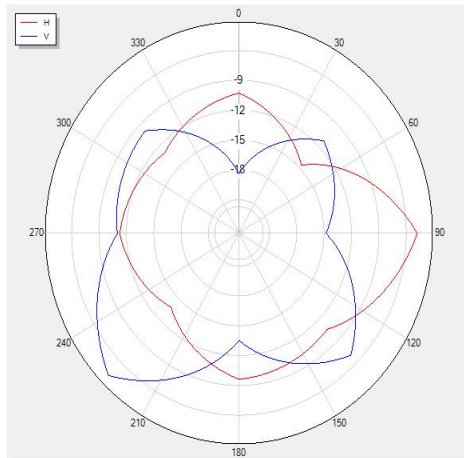
2450 Polar
