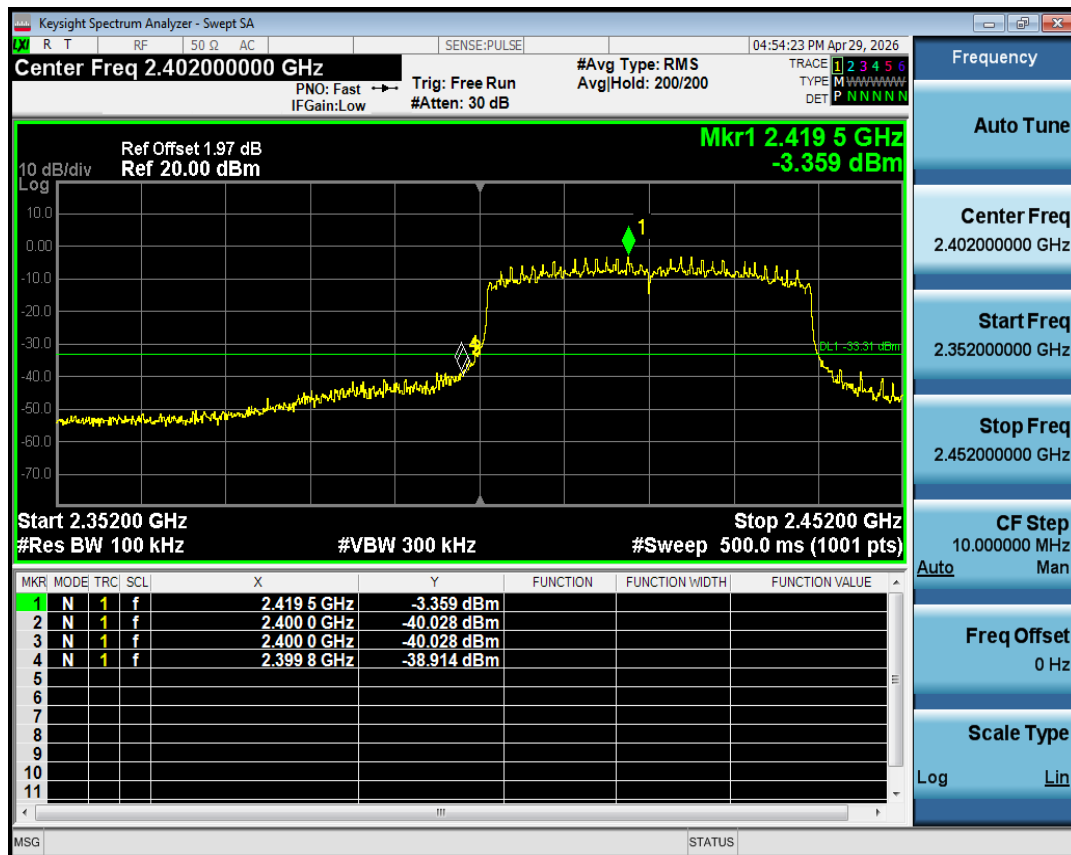
Band Edge NVNT ax40 2422MHz Ant1 Emission
