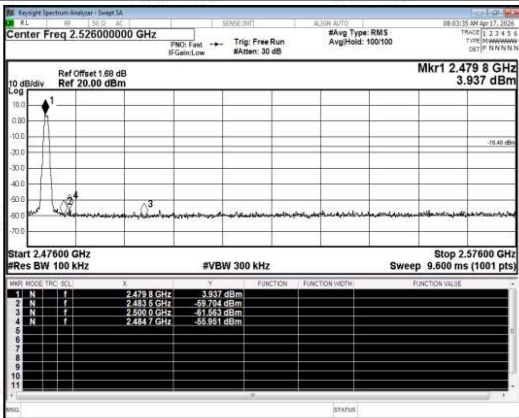
Band Edge NVNT BLE 2480MHz Ant1 Emission
