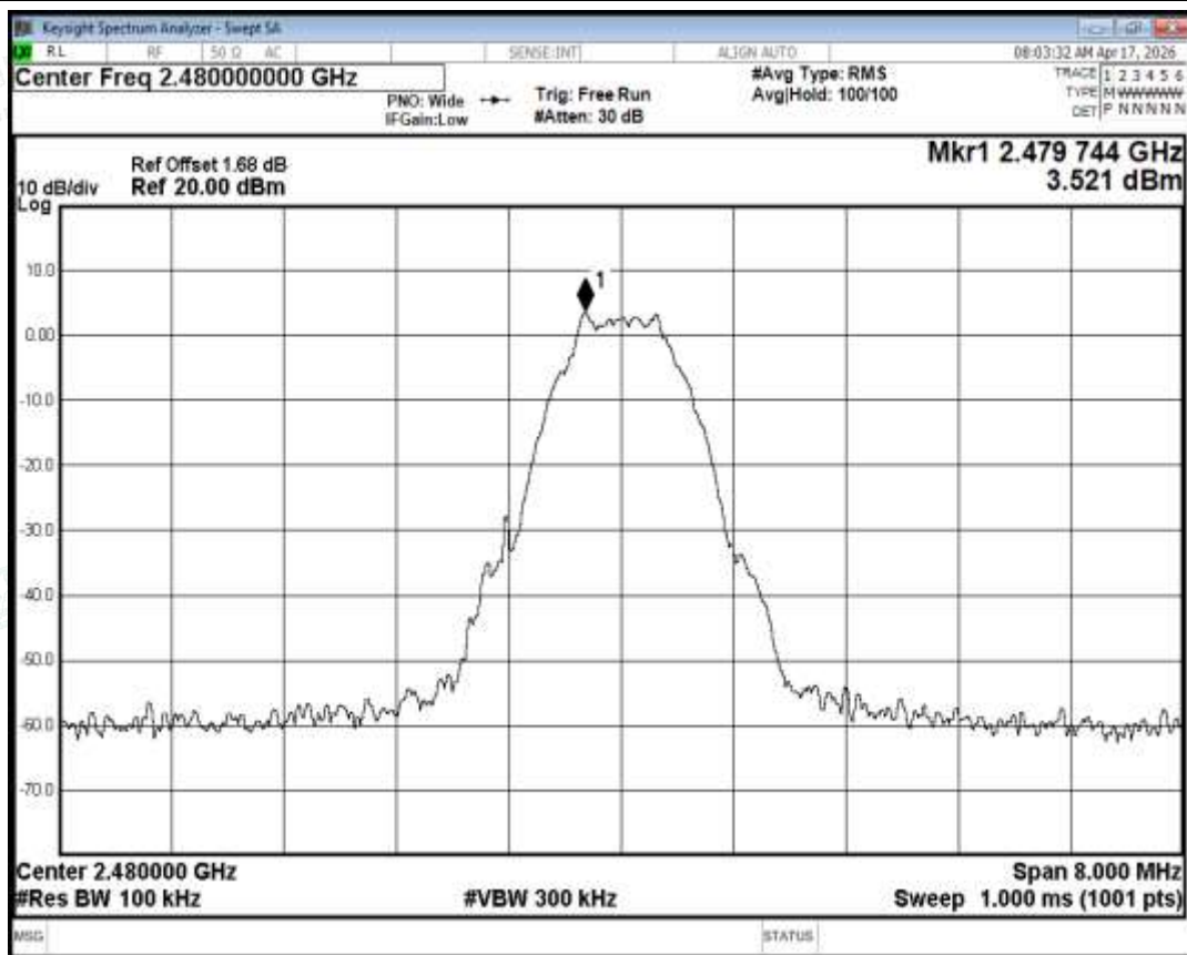
Band Edge NVNT BLE 2480MHz Ant1 Ref
