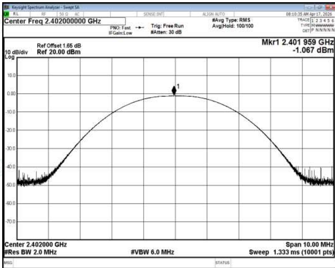
Peak Power NVNT BLE 2402MHz Ant1
