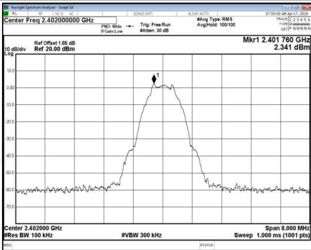
Band Edge NVNT BLE 2402MHz Ant1 Ref
