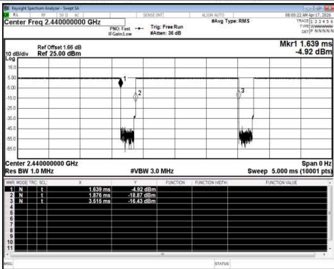
Duty Cycle NVNT BLE 2440MHz Ant1
