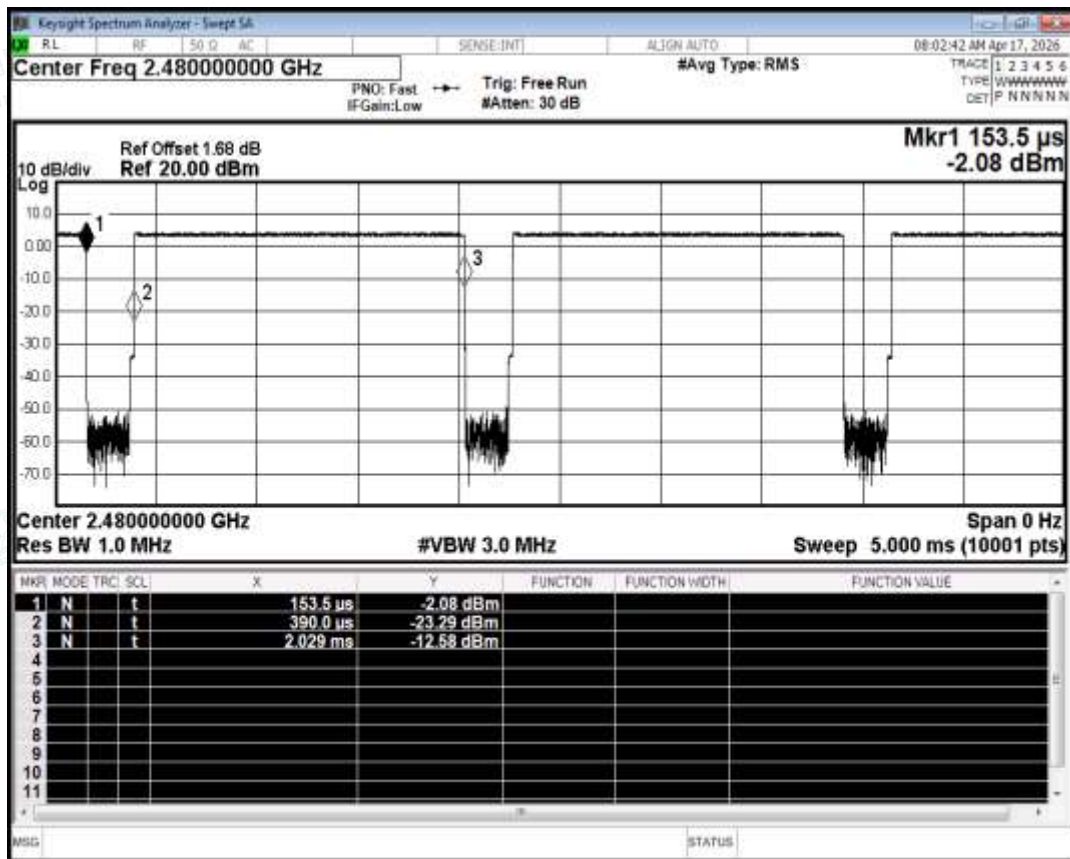
Duty Cycle NVNT BLE 2480MHz Ant1
