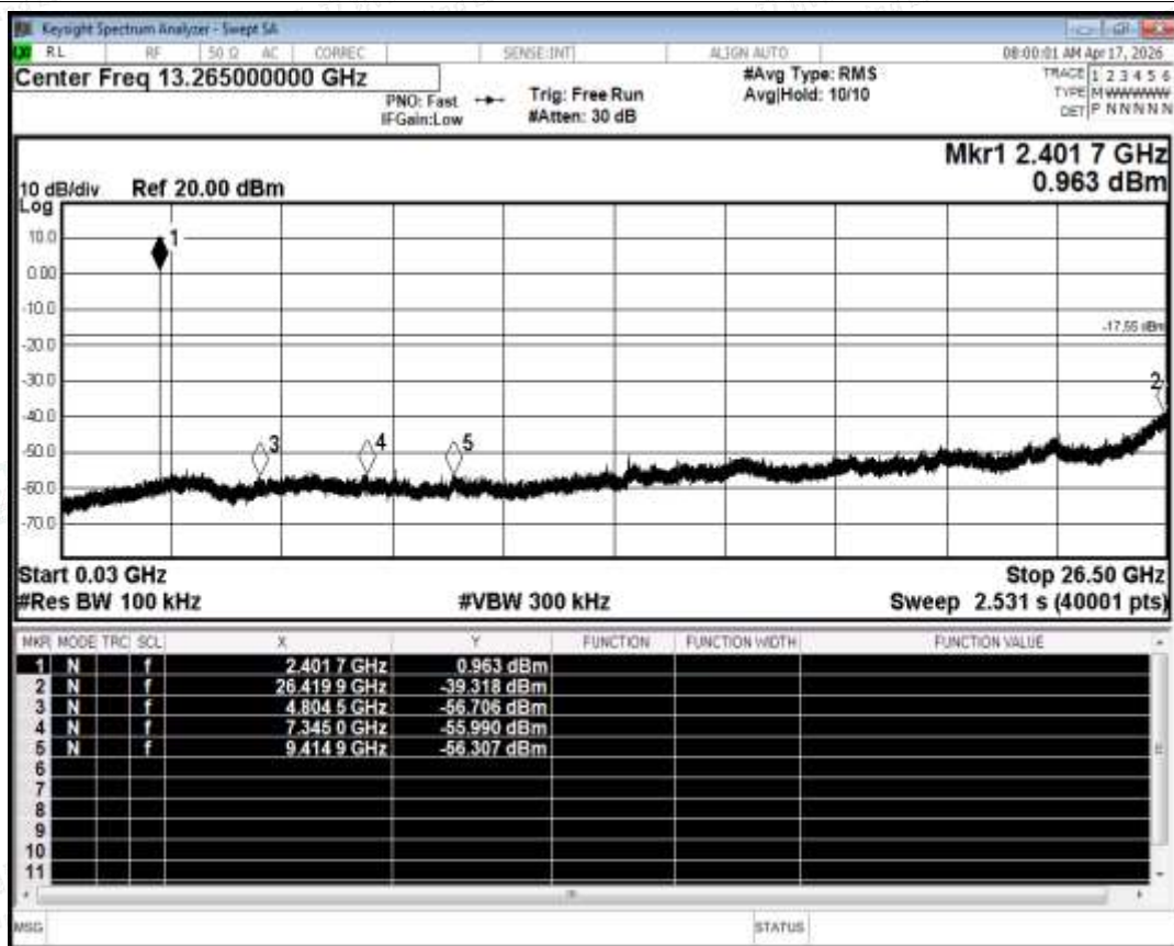
Tx. Spurious NVNT BLE 2402MHz Ant1 Emission
