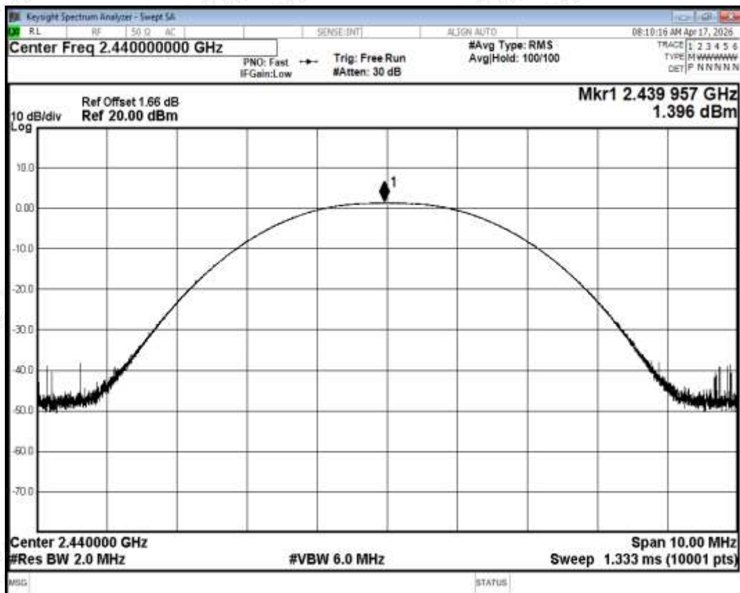
Peak Power NVNT BLE 2440MHz Ant1
