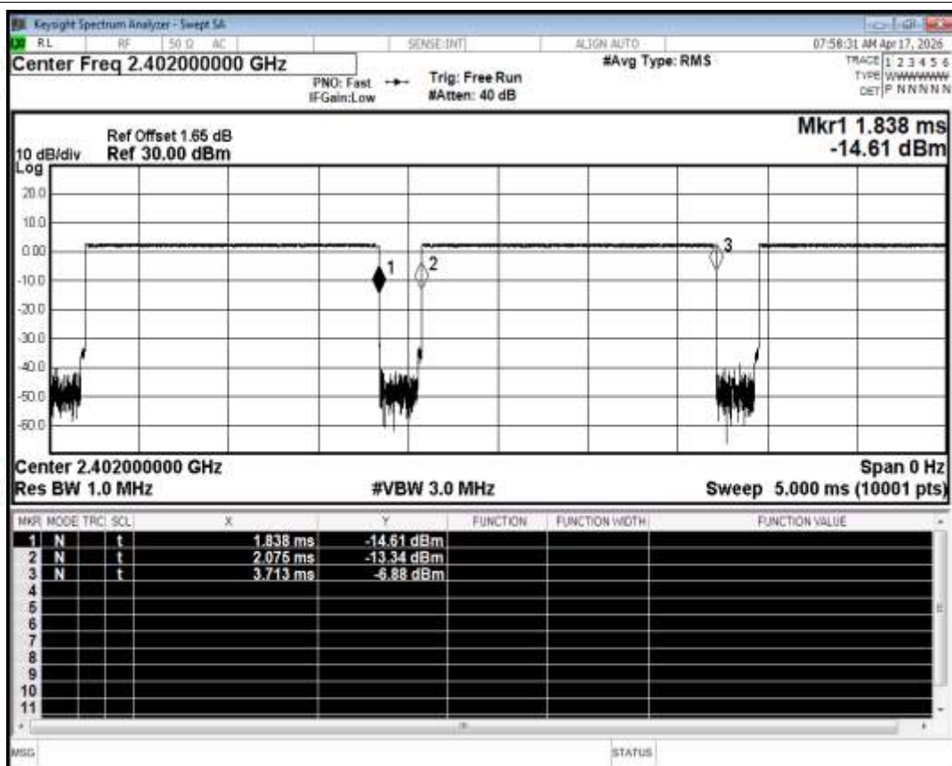
Duty Cycle NVNT BLE 2402MHz Ant1
