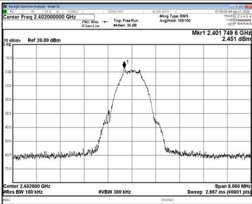
Tx. Spurious NVNT BLE 2402MHz Ant1 Ref
