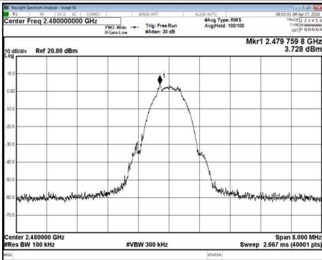
Tx. Spurious NVNT BLE 2480MHz Ant1 Ref
