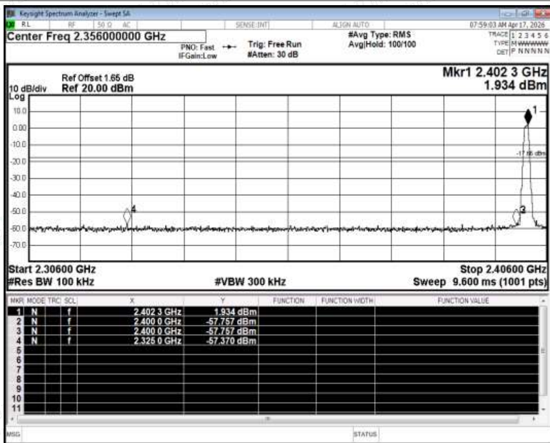
Band Edge NVNT BLE 2402MHz Ant1 Emission
