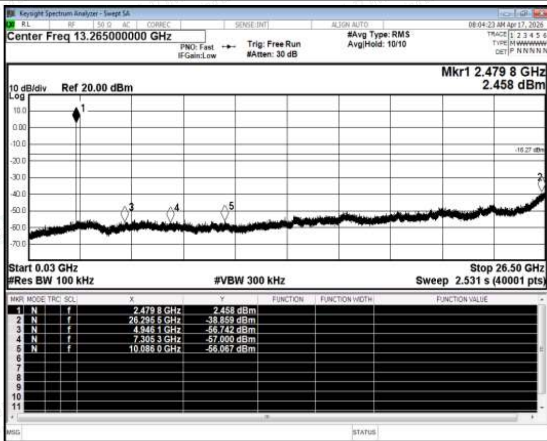
Tx. Spurious NVNT BLE 2480MHz Ant1 Emission
