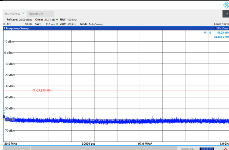
11G-Ant1-2412-30~1000-PASS
