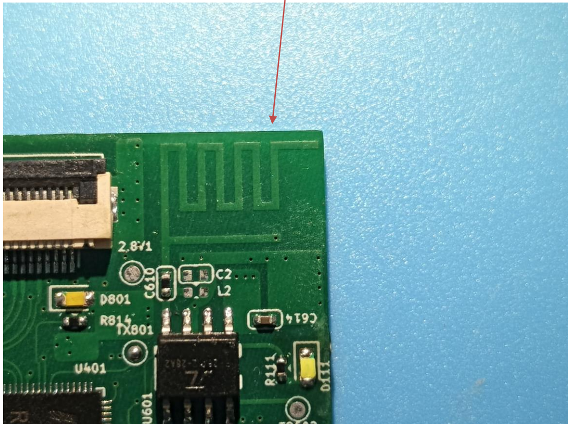
Antenna
