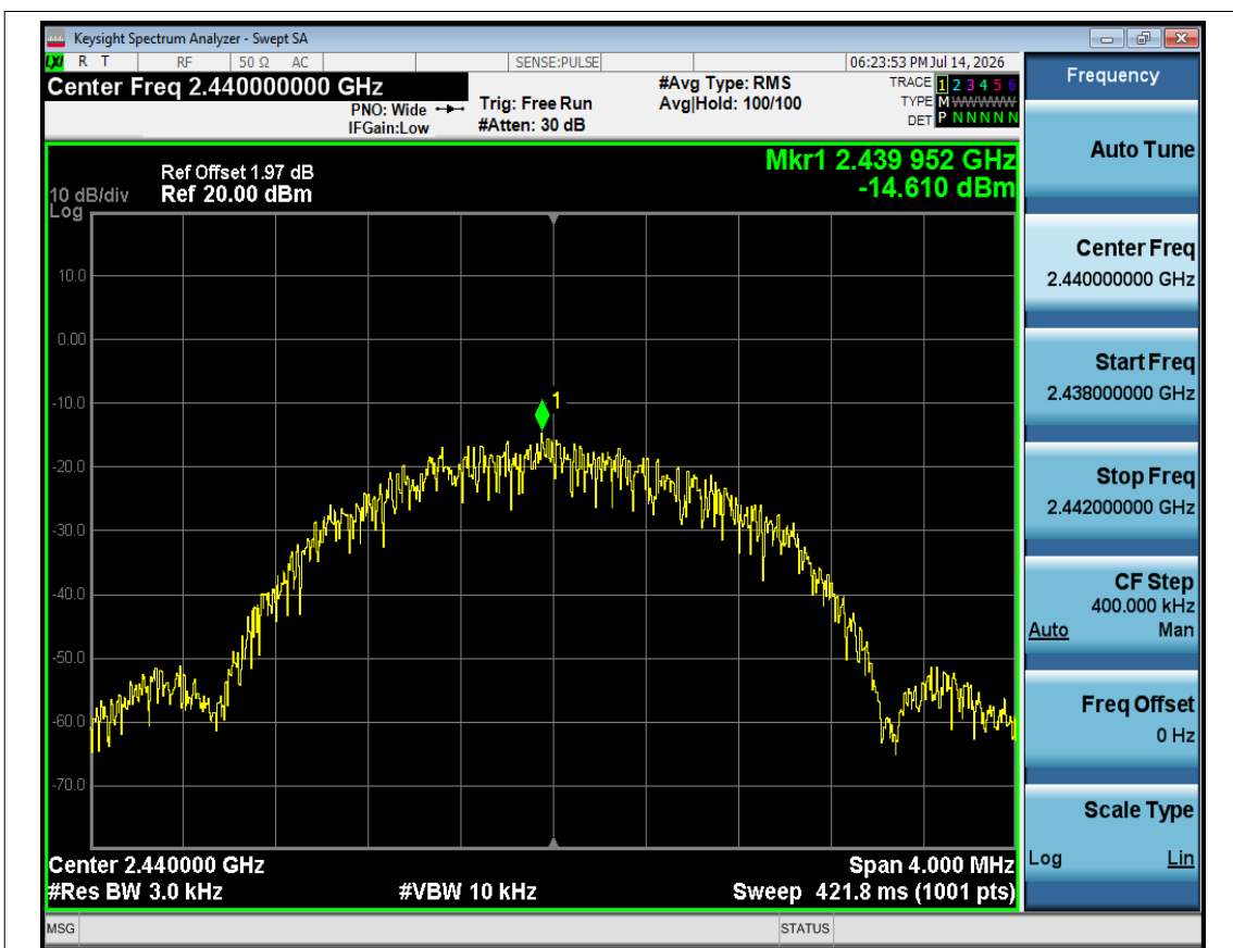
PSD NVNT BLE 2M 2440MHz Ant1
