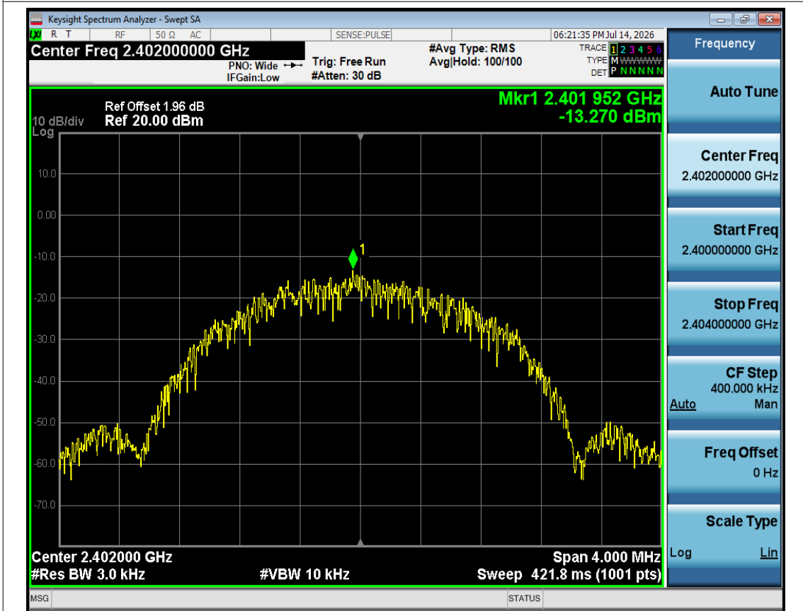
PSD NVNT BLE 2M 2402MHz Ant1
