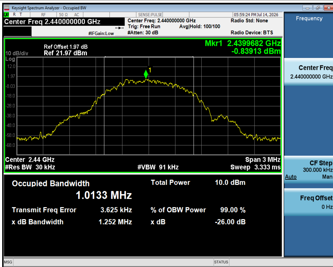
OBW NVNT BLE 1M 2440MHz Ant1
