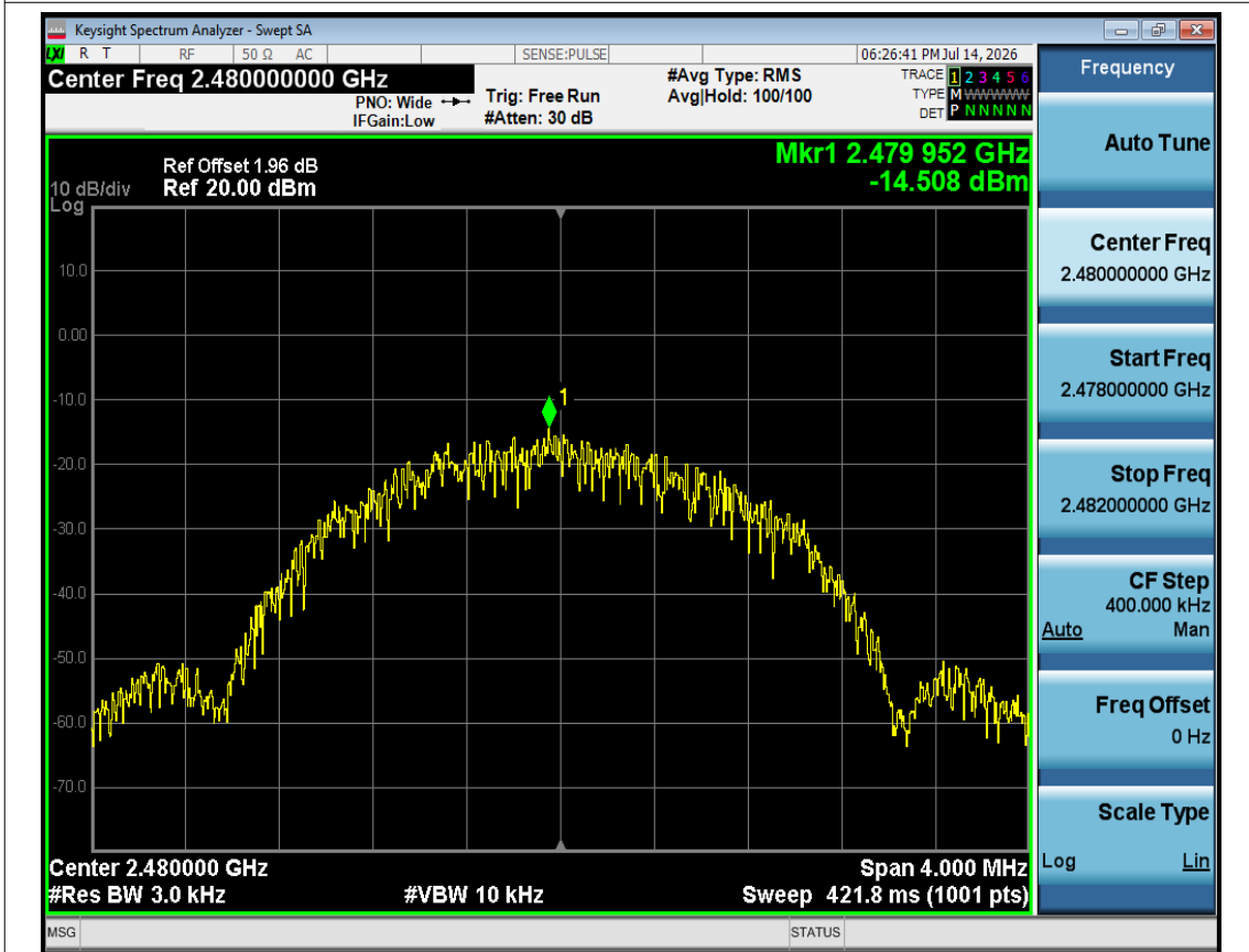
PSD NVNT BLE 2M 2480MHz Ant1
