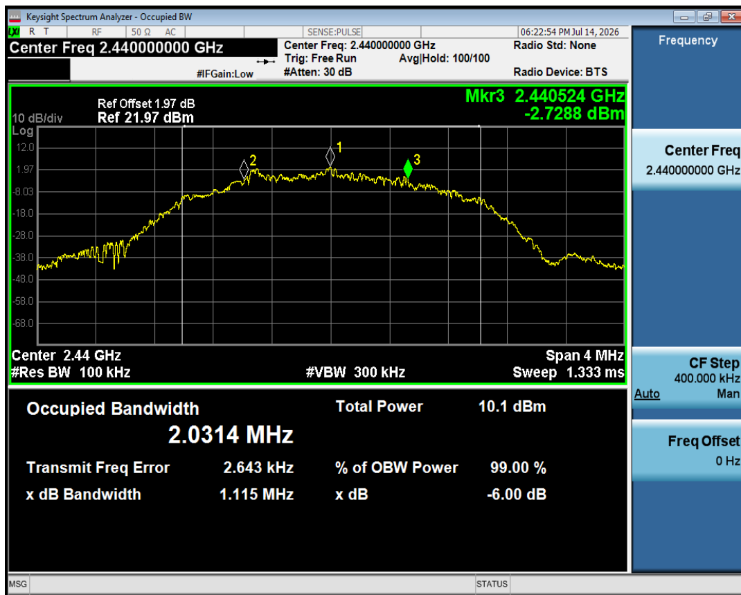
-6dB Bandwidth NVNT BLE 2M 2440MHz Ant1
