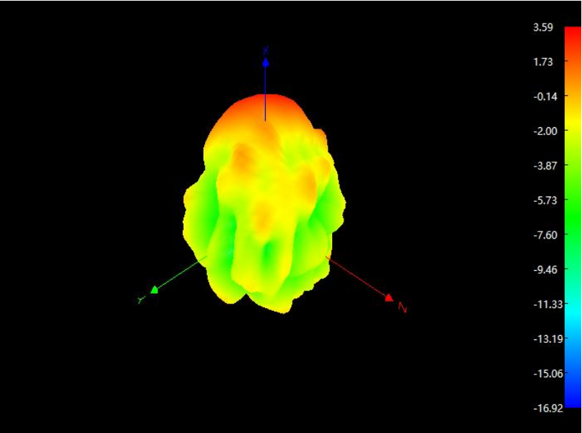
天线辐射方向图 Antenna Radiation Patterns
