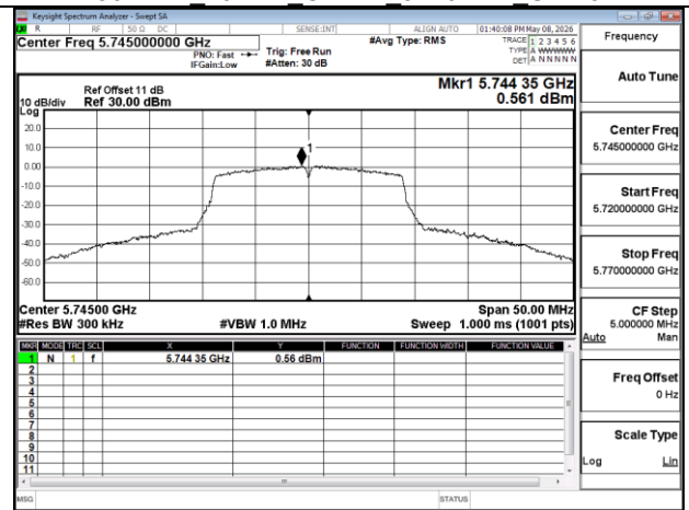
802.11n 20MHz Chain1 5745MHz
