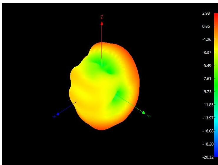
2450MHz 3D
