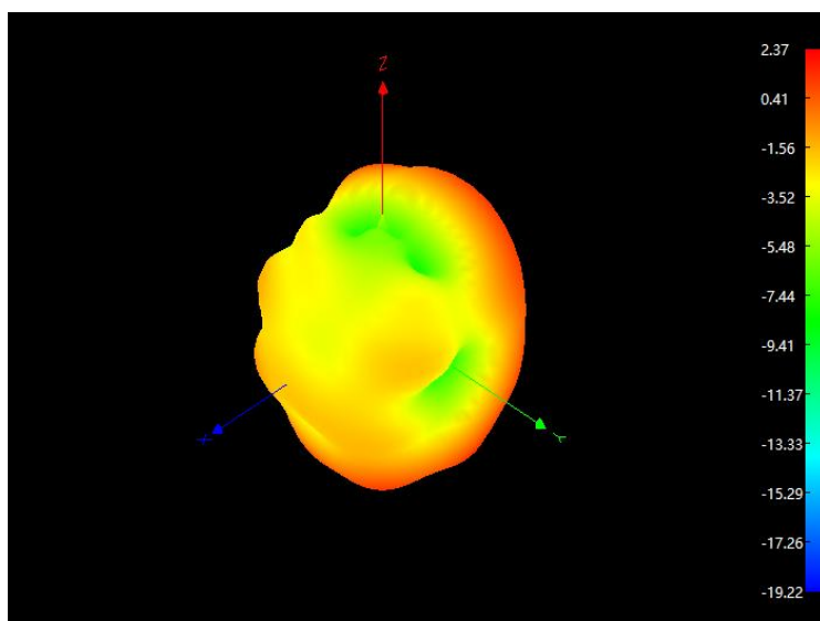
2500MHz 3D
