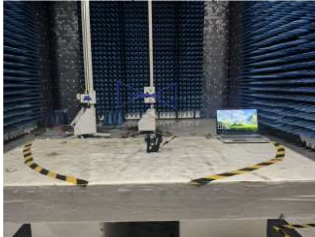
RE (Below 1GHz)
