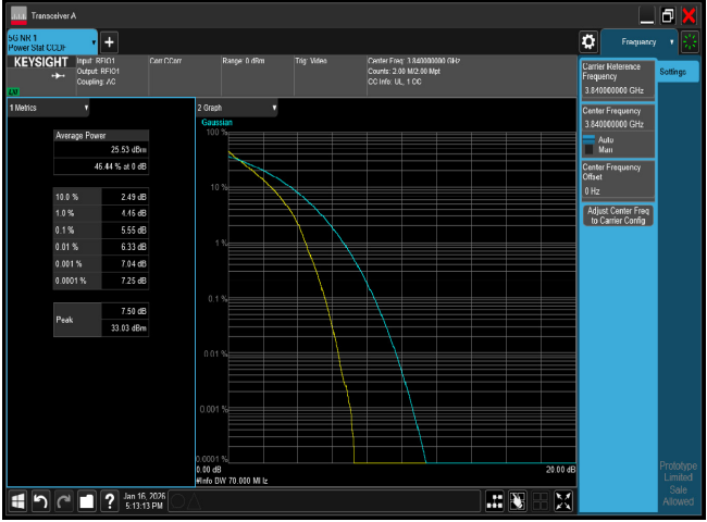
PTAR B77 70M CH656000 QPSK
