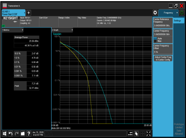
PTAR B77 60M CH656000 QPSK
