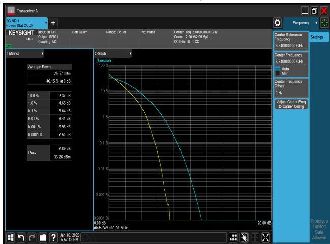
PTAR B77 100M CH656000 QPSK
