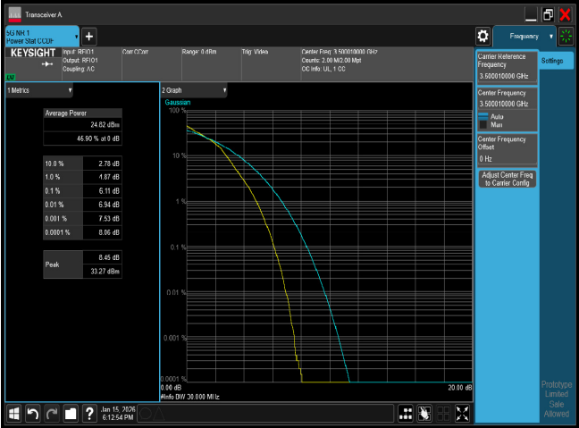
PTAR n77 30M CH633334 16QAM
