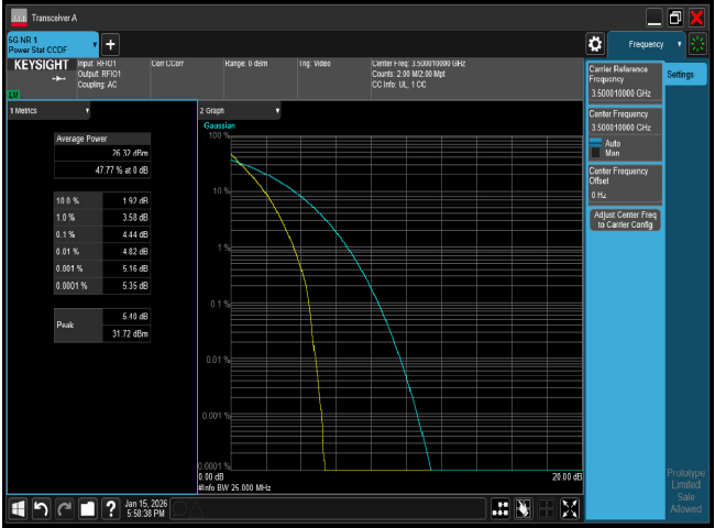
PTAR n77 25M CH633334 BPSK
