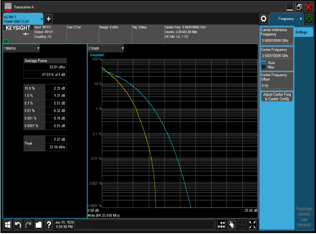
PTAR n77 25M CH633334 QPSK
