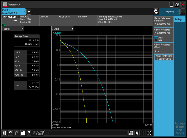
PTAR n77 30M CH633334 BPSK
