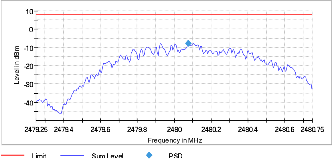
Power Spectral Densitiv (AVGPSD-3)
