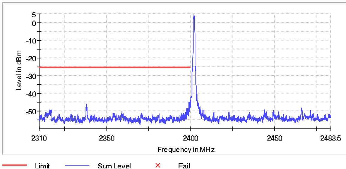
Band Edge
