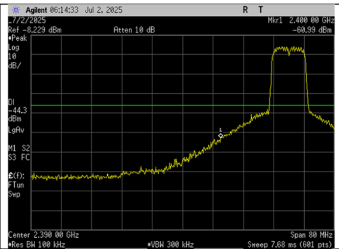
Low Ch_2418MHz_10MHz BW_-30dBc_Lower Band Edge Port 2
