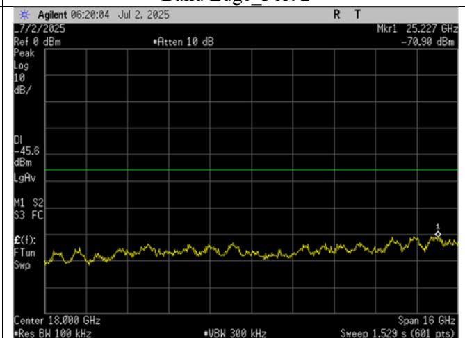
High Ch_2457MHz_10MHz BW_-30dBc_10- 26GHz_Port 2
