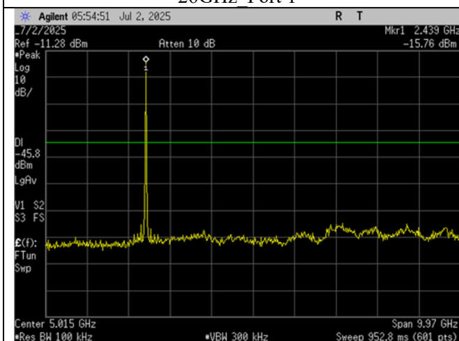
Mid Ch_2440MHz_10MHz BW_-30dBc_30MHz- 10GHz Port 1
