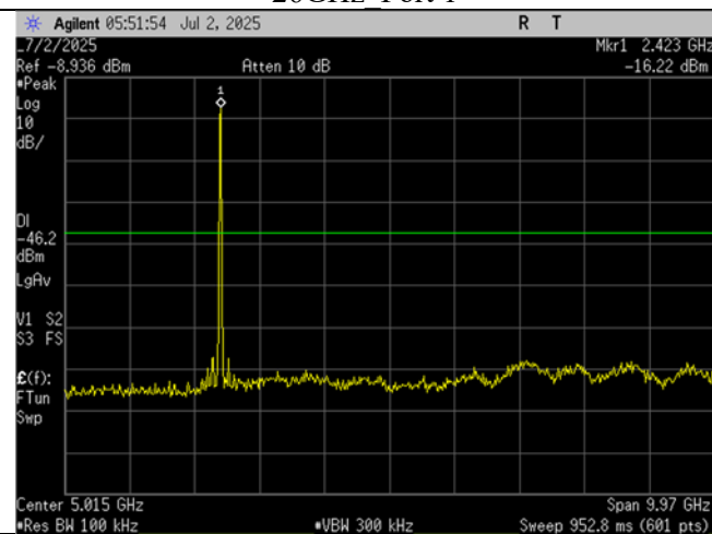
Low Ch_2418MHz_10MHz BW_-30dBc_30MHz-10GHz Port 1
