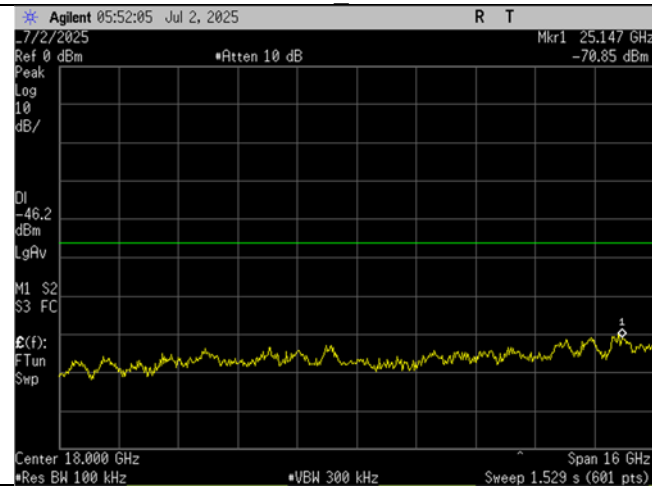
Low Ch_2418MHz_10MHz BW_-30dBc_10-26GHz Port 1
